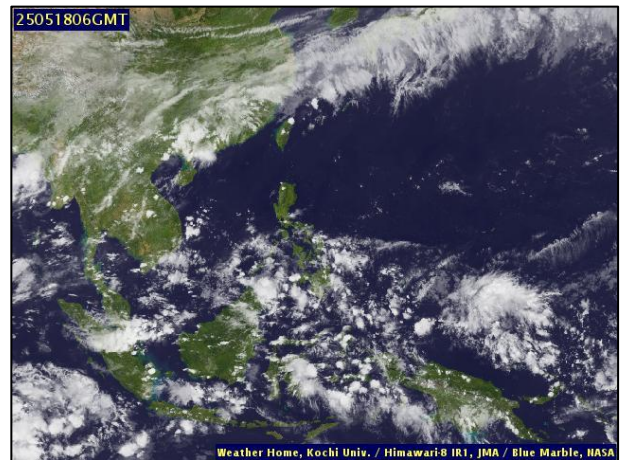
ภาพถ่ายดาวเทียม วันที่ ๑๘ พ.ค. ๒๕๖๘ เวลา ๑๓.๐๐ น.
