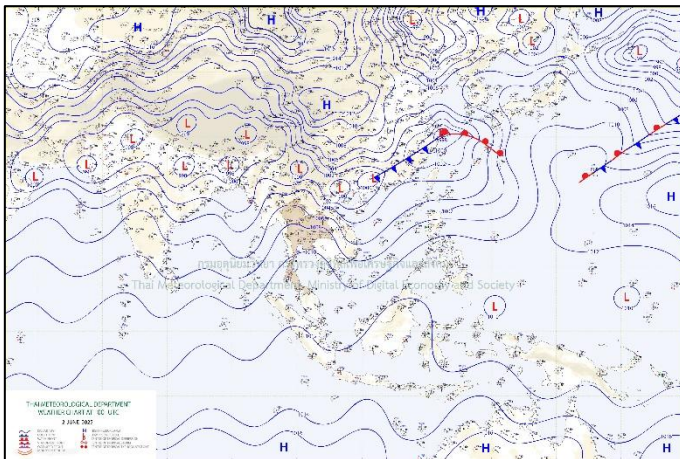
แผนที่อากาศ วันที่ ๒ มิ.ย. ๒๕๖๘ เวลา ๐๗.๐๐ น.
