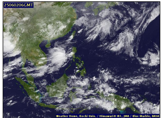
ภาพถ่ายดาวเทียม วันที่ ๒ มิ.ย. ๒๕๖๘ เวลา ๑๓.๐๐ น.
