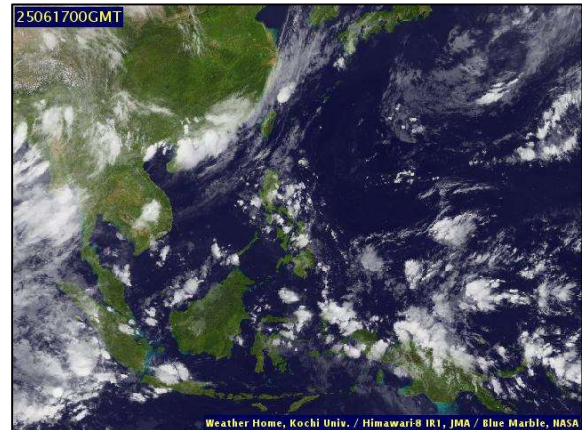
ภาพถ่ายดาวเทียม วันที่ ๑๗ มิ.ย. ๒๕๖๘ เวลา ๐๗.๐๐ น.
