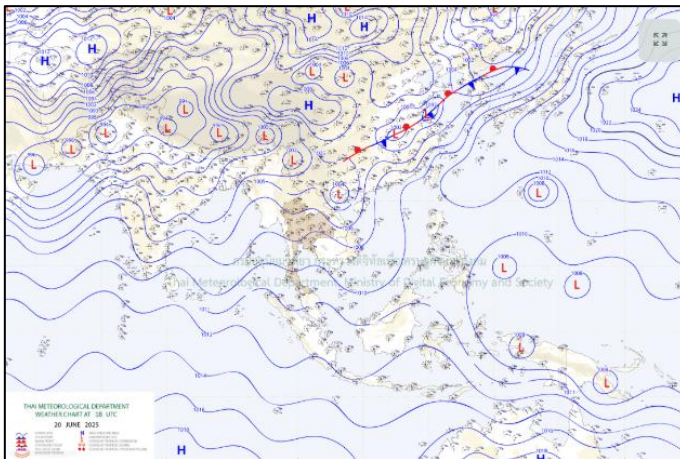
แผนที่อากาศ วันที่ ๒๑ มิ.ย. ๒๕๖๘ เวลา ๐๑.๐๐ น.
