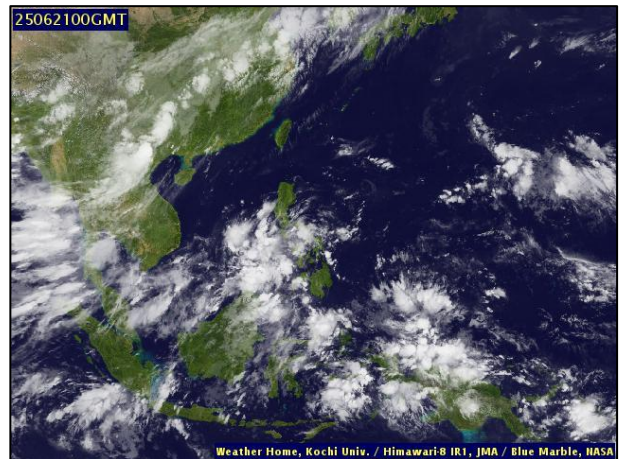
ภาพถ่ายดาวเทียม วันที่ ๒๑ มิ.ย. ๒๕๖๘ เวลา ๐๗.๐๐ น.
