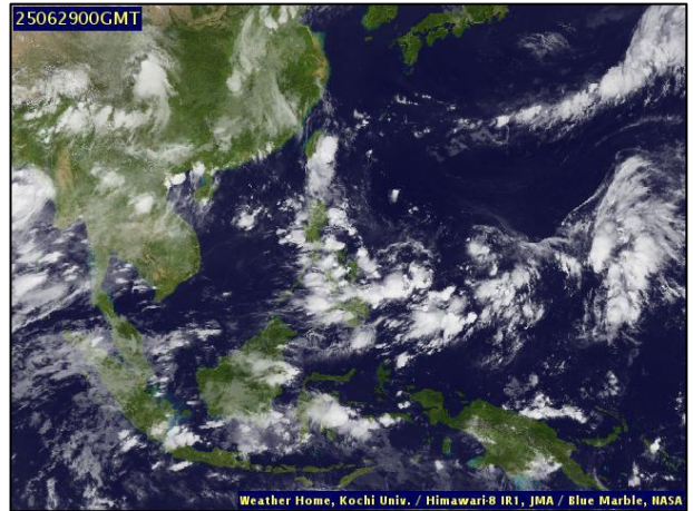
ภาพถ่ายดาวเทียม วันที่ ๒๙ มิ.ย. ๒๕๖๘ เวลา ๐๗.๐๐ น.
