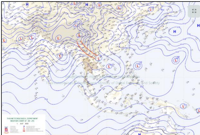
แผนที่อากาศ วันที่ ๑ ก.ค. ๒๕๖๘ เวลา ๐๗.๐๐ น.
