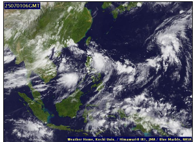
ภาพถ่ายดาวเทียม วันที่ ๑ ก.ค. ๒๕๖๘ เวลา ๑๓.๐๐ น.
