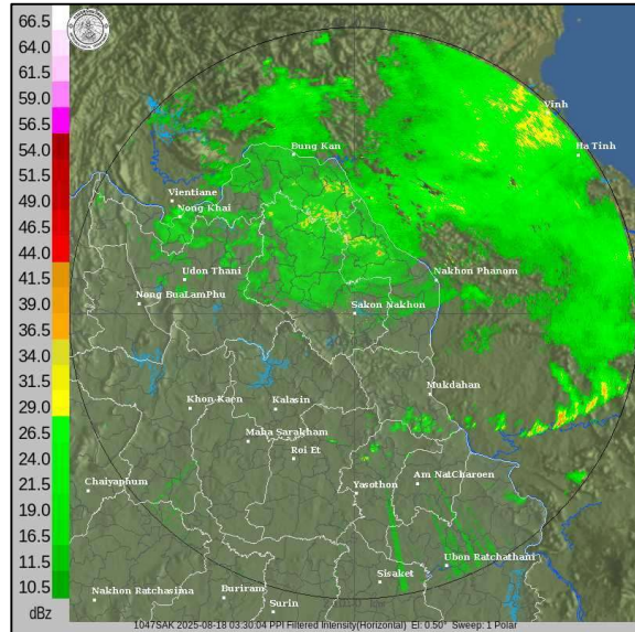
สถานีสกลนคร เวลา ๑๐.๓๐ น.
