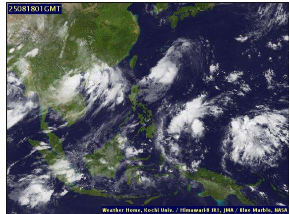
ภาพถ่ายดาวเทียม วันที่ ๑๘ ส.ค. ๒๕๖๘ เวลา ๐๘.๐๐ น.
