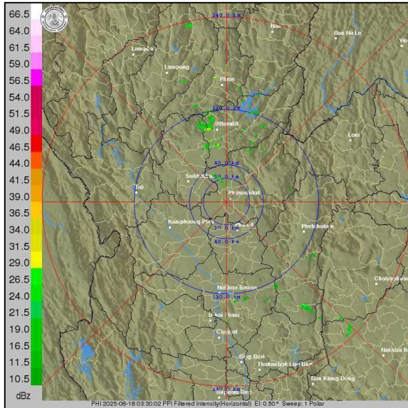
สถานีพิษณุโลก ๑๐.๓๐ น.
