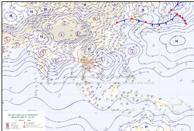
แผนที่อากาศ วันที่ ๑๘ ส.ค. ๒๕๖๘ เวลา ๐๑.๐๐ น.
