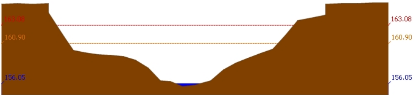
สถานี 120105T แม่น้ำป่าสักที่บ้านวังมเหนือ ต.ทำอัญญา อ.หล่มสัก จ.เพชรบูรณ์ ระดับน้ำ 156.05 ม.รทก.
