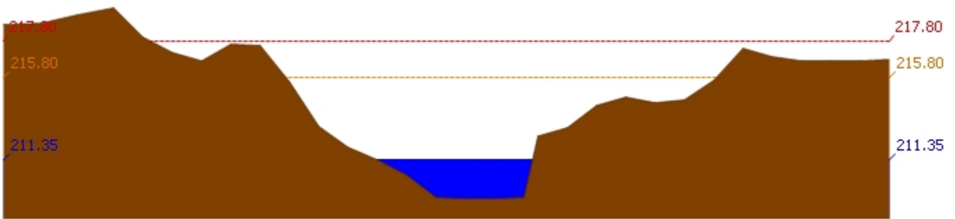
สถานี 120205T แม่น้ำป่าสักที่บ้านอู่กะทาด ต.ศิลา อ.หล่มเก่า จ.เพชรบูรณ์ ระดับน้ำ 211.35 ม.รทก.
