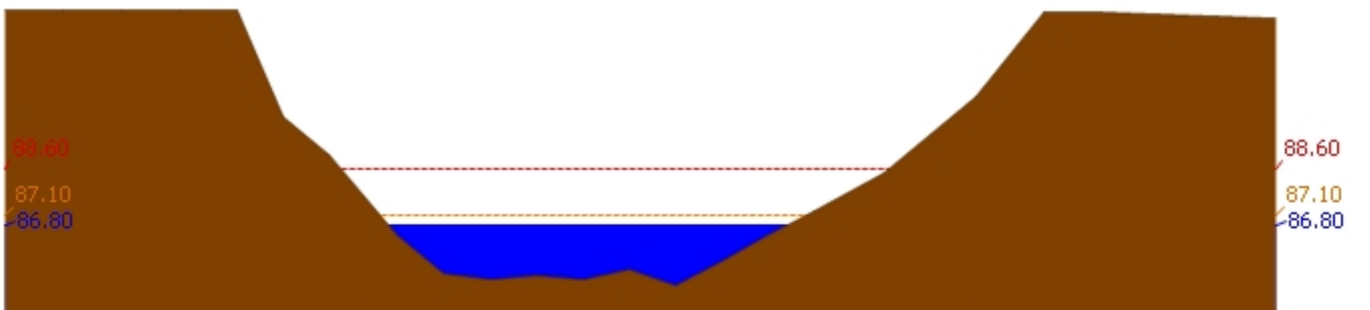
สถานี 120110T แม่น้ำป่าสักที่บ้านวังโบสถ์ ต.วังโบสถ์ อ.หนองไผ่ จ.เพชรบูรณ์ ระดับน้ำ 86.80 ม.รทก.
