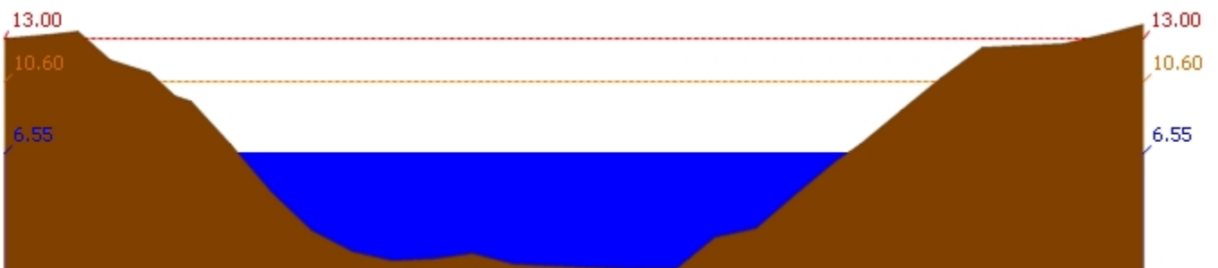
สถานี 120106T แม่น้ำป่าสักที่ อ.เสนาห์ ต.ศาลาวิไทย อ.เสนาห์ จ.สระบุรี ระดับน้ำ 6.55 ม.รทก.
