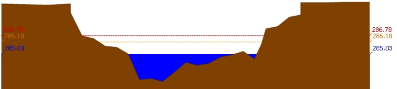
สถานี 070111T แม่น้ำวังที่บ้านแปงโปงชัย ต.บ้านเสา อ.แจ้ห่ม จ.ลำปาง ระดับน้ำ 285.03 ม.รทก.
