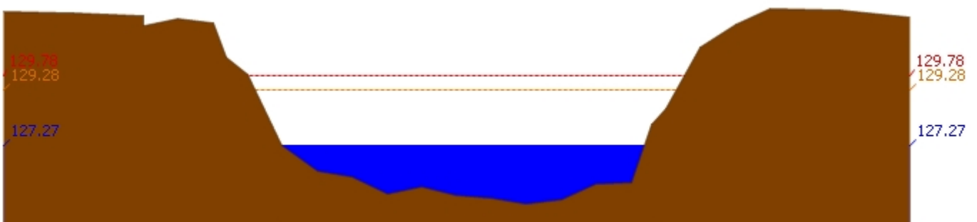
สถานี 070118T แม่น้ำวังที่บ้านแม่สลิด ต.แม่สลิด อ.บ้านตาก จ.ตาก ระดับน้ำ 127.27 ม.รทก.
