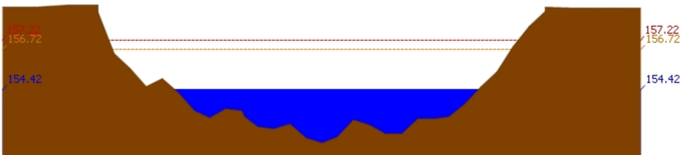
สถานี 070117T แม่น้ำวังที่เทศบาลตำบลแม่ปู้ ต.แม่ปู้ อ.แม่พริก จ.ลำปาง ระดับน้ำ 154.42 ม.รทก.
