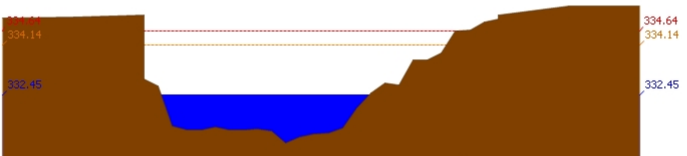
สถานี 070304T น้ำแม่สอยที่บ้านหนองกอก ต.แม่สุก อ.แจ้ห่ม จ.ลำปาง ระดับน้ำ 332.45 ม.รทก.
