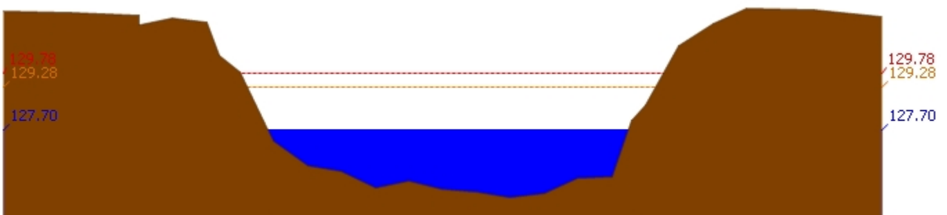
สถานี 070118T แม่น้ำวังที่บ้านแม่สลิด ต.แม่สลิด อ.บ้านตาก จ.ตาก ระดับน้ำ 127.70 ม.รทก.
