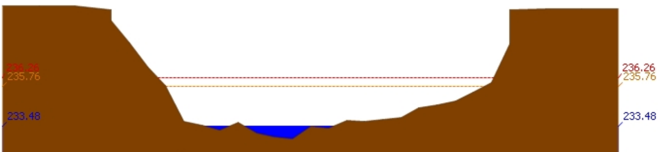
สถานี 070114T แม่น้ำวังที่บ้านปงชัย ต.บ้านเสด็จ อ.เมืองลำปาง จ.ลำปาง ระดับน้ำ 233.48 ม.รทก.
