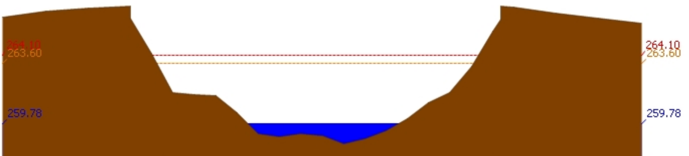
สถานี 070112T แม่น้ำวังที่บ้านบุญนาต ต.บุญนาตพัฒนา อ.เมืองลำปาง จ.ลำปาง ระดับน้ำ 259.78 ม.รทก.
