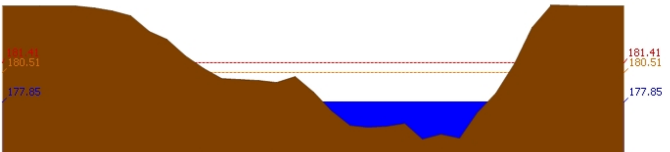
สถานี 070116T แม่น้ำวังที่บ้านแม่เตี๊ยะ ต.แม่ถอด อ.เถิน จ.ลำปาง ระดับน้ำ 177.85 ม.รทก.
