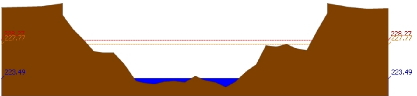
สถานี 070113T แม่น้ำวังที่ จ.ลำปาง ต.เวียงเหนือ อ.เมืองลำปาง จ.ลำปาง ระดับน้ำ 223.49 ม.รทก.
