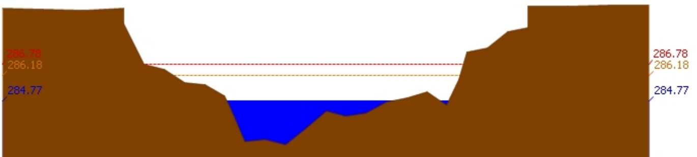
สถานี 070111T แม่น้ำวังที่บ้านแปงโปงชัย ต.บ้านเสา อ.แจ้ห่ม จ.ลำปาง ระดับน้ำ 284.77 ม.รทก.
