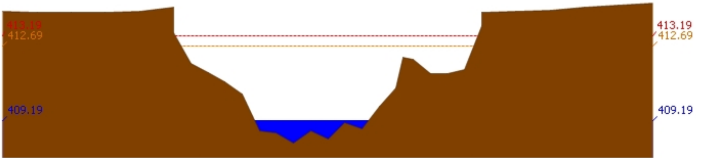
สถานี 070110T แม่น้ำวังที่ อ.วังเหนือ ต.วังเหนือ อ.วังเหนือ จ.ลำปาง ระดับน้ำ 409.19 ม.รทก.
