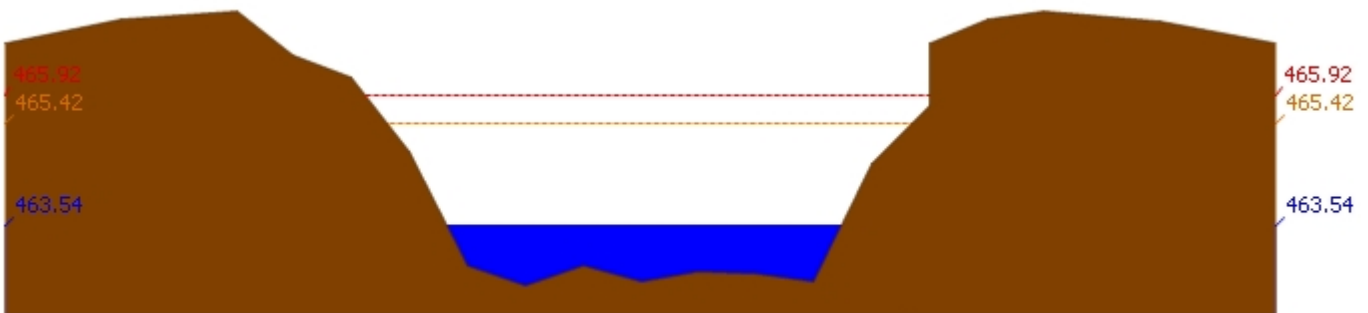
สถานี 061206T น้ำแม่แจ่มที่บ้านทัพ ต.ท่าผา อ.แม่แจ่ม จ.เชียงใหม่ ระดับน้ำ 463.54 ม.รทก.
