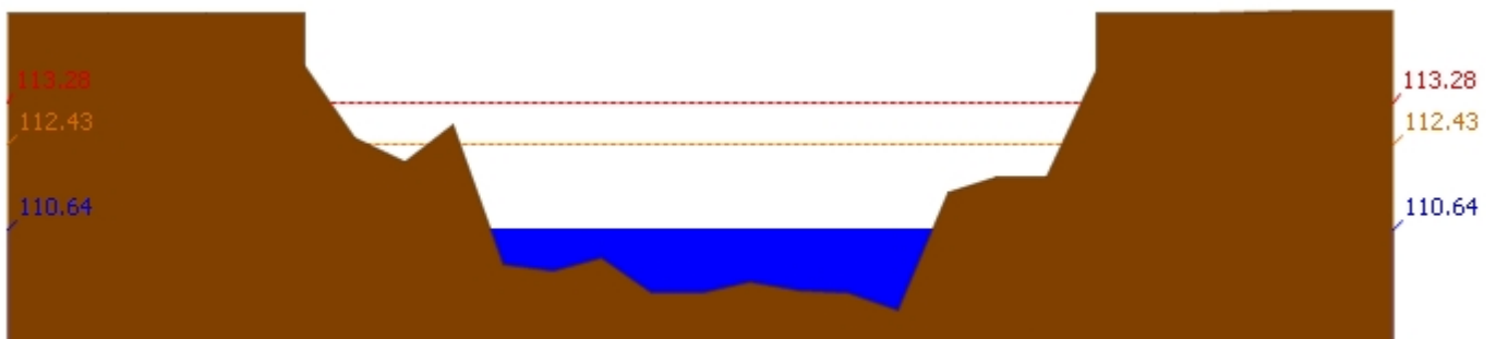
สถานี 061801T คลองวังเจ้าที่บ้านคลองลึก ต.เชิงทอง อ.วังเจ้า จ.ตาก ระดับน้ำ 110.64 ม.รทก.
