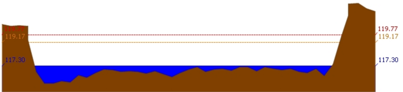
สถานี 060111T แม่น้ำปิงที่บ้านปากร่องห้วยจี่ ต.ตากออก อ.บ้านตาก จ.ตาก ระดับน้ำ 117.30 ม.รทก.
