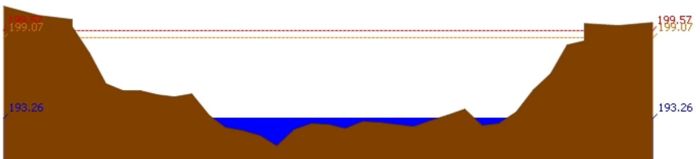
สถานี 070115T น้ำแม่วังที่บ้านอ้อ ต.แม่กัวะ อ.สบปราบ จ.ลำปาง ระดับน้ำ 193.26 ม.รทก.
