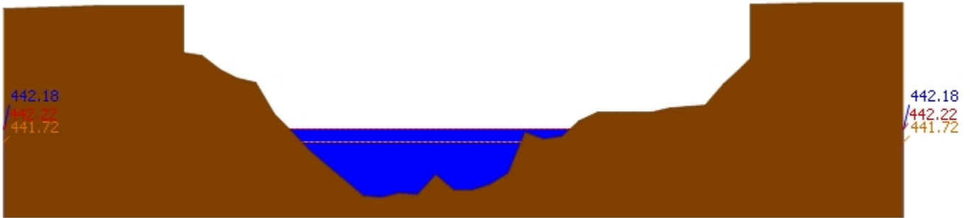
สถานี 060905T น้ำแม่สีที่อำเภอสีคิ้ว อ.สีคิ้ว จ.ลำพูน ระดับน้ำ 442.18 ม.รทก.
