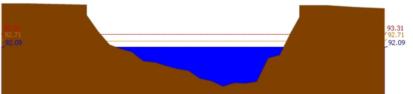
สถานี 061901T คลองแม่ระกาที่บ้านวังชะโอน ต.ท่าไม้ อ.พรานกระต่าย จ.กำแพงเพชร ระดับน้ำ 92.09 ม.รทก.
