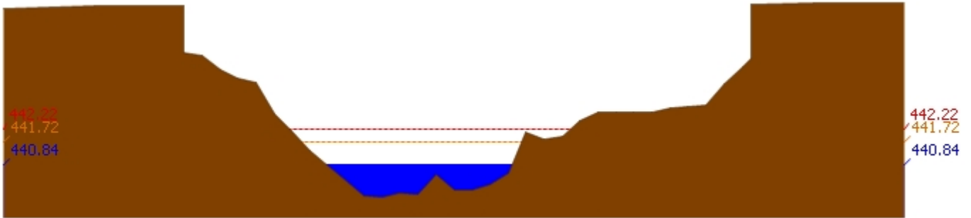
สถานี 060905T น้ำแม่ลี้ที่อำเภอลี้ ต.ลี้ อ.ลี้ จ.ลำพูน ระดับน้ำ 440.84 ม.รทก.
