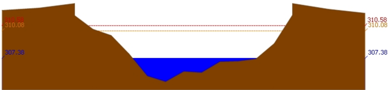
สถานี 060814T น้ำแม่ขานที่บ้านท่าโป่ง ต.บ้านแม อ.สันป่าตอง จ.เชียงใหม่ ระดับน้ำ 307.38 ม.รทก.
