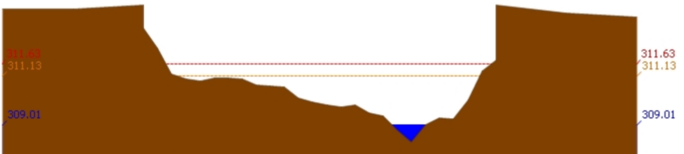
สถานี 061401T น้ำแม่หาดที่บ้านโป่งทุ่ง ต.โป่งทุ่ง อ.คอยเต่า จ.เชียงใหม่ ระดับน้ำ 309.01 ม.รทก.
