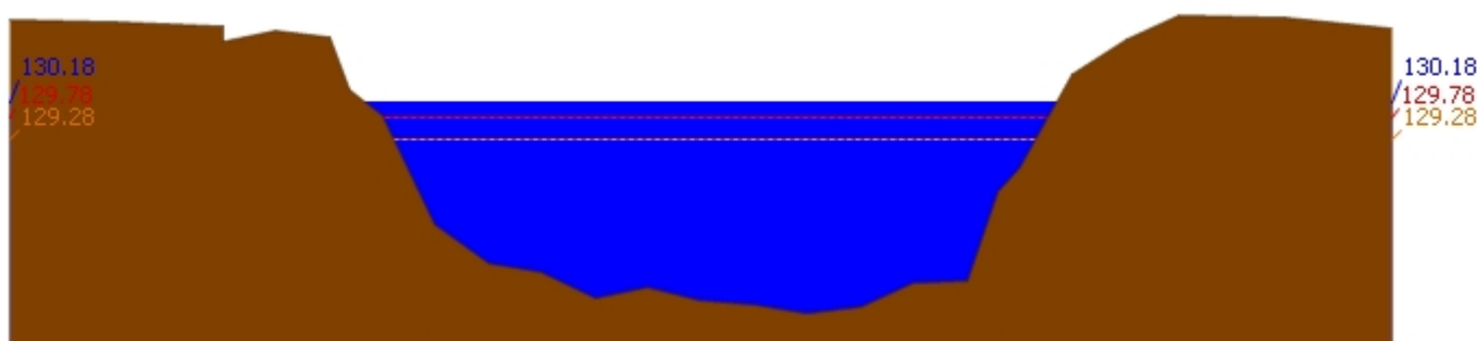
สถานี 070118T แม่น้ำวังที่บ้านแม่สลิด ต.แม่สลิด อ.บ้านตาก จ.ตาก ระดับน้ำ 130.18 ม.รทก.
