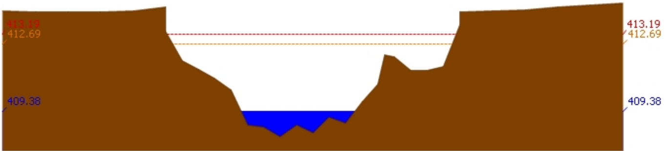
สถานี 070110T แม่น้ำวังที่ อ.วังเหนือ ต.วังเหนือ อ.วังเหนือ จ.ลำปาง ระดับน้ำ 409.38 ม.รทก.
