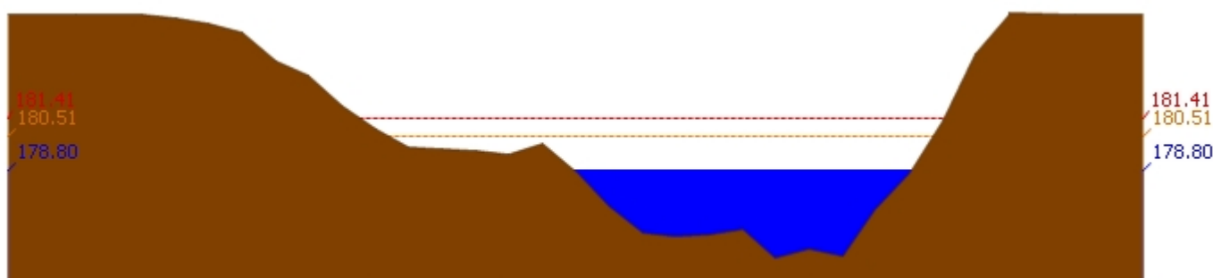
สถานี 070116T แม่น้ำวังที่บ้านแม่เตี๊ยะ ต.แม่ถอด อ.เถิน จ.ลำปาง ระดับน้ำ 178.80 ม.รทก.
