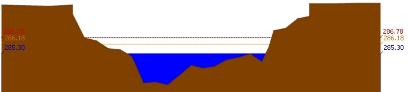
สถานี 070111T แม่น้ำวังที่บ้านแปงโปงชัย ต.บ้านเสา อ.แจ้ห่ม จ.ลำปาง ระดับน้ำ 285.30 ม.รทก.
