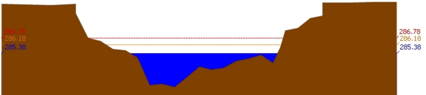
สถานี 070111T แม่น้ำวังที่บ้านแปงโปงชัย ต.บ้านเสา อ.แจ้ห่ม จ.ลำปาง ระดับน้ำ 285.38 ม.รทก.
