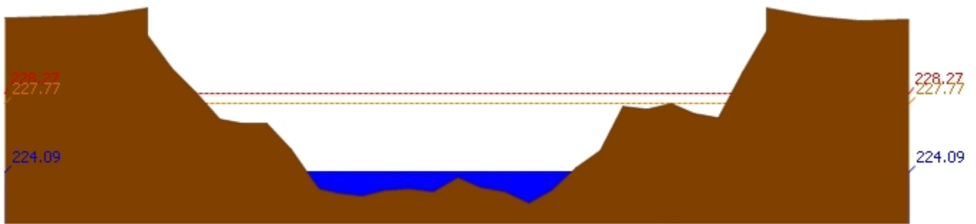
สถานี 070113T แม่น้ำวังที่ จ.ลำปาง ต.เวียงเหนือ อ.เมืองลำปาง จ.ลำปาง ระดับน้ำ 224.09 ม.รทก.
