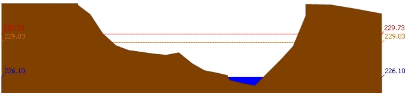
สถานี 070703T น้ำแม่ต่ำที่บ้านนาบอน ต.ทุ่งงาม อ.เสริมงาม จ.ลำปาง ระดับน้ำ 226.10 ม.รทก.
