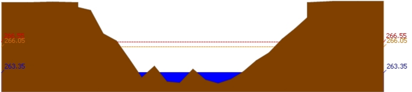
สถานี 070604T น้ำแม่จางที่บ้านสุโหมไชยมงคล ต.หัวเสือ อ.แม่ทะ จ.ลำปาง ระดับน้ำ 263.35 ม.รทก.
