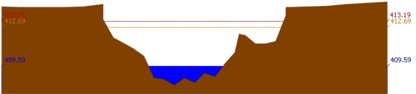
สถานี 070110T แม่น้ำวังที่ อ.วังเหนือ ต.วังเหนือ อ.วังเหนือ จ.ลำปาง ระดับน้ำ 409.59 ม.รทก.
