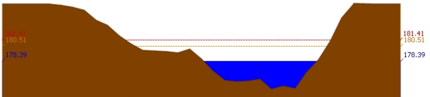
สถานี 070116T แม่น้ำวังที่บ้านแม่เตี๊ยะ ต.แม่ถอด อ.เถิน จ.ลำปาง ระดับน้ำ 178.39 ม.รทก.
