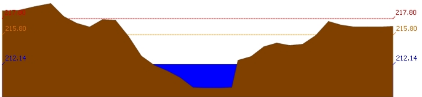
สถานี 120205T แม่น้ำป่าสักที่บ้านอู่กระทาด ต.ศิลา อ.หล่มเก่า จ.เพชรบูรณ์ ระดับน้ำ 212.14 ม.รทก.
