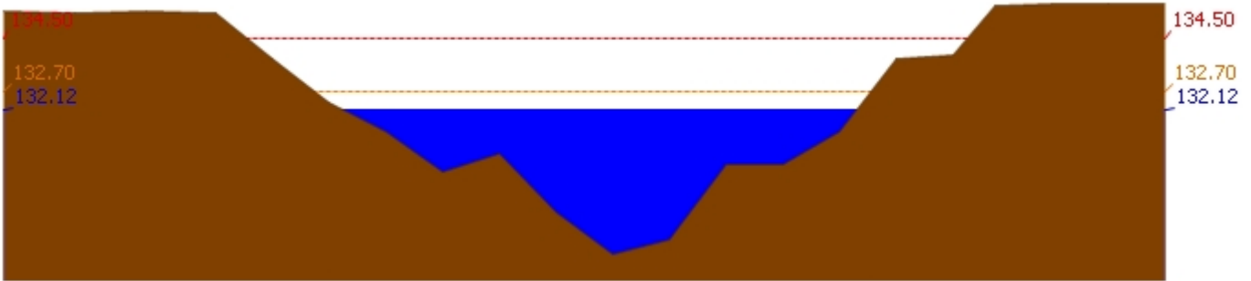
สถานี 120111T แม่น้ำป่าสักที่บ้านจางวาง ต.ลานบัว อ.หล่มสัก จ.เพชรบูรณ์ ระดับน้ำ 132.12 ม.รทก.
