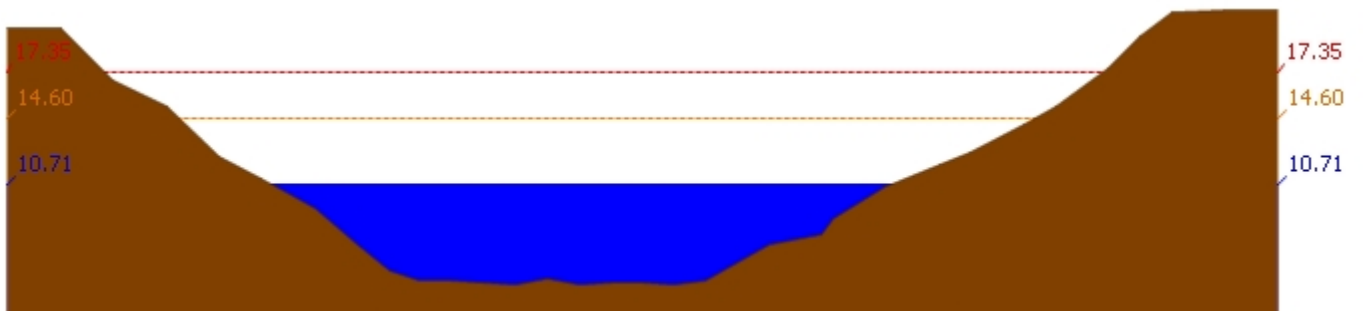
สถานี 120109T แม่น้ำป่าสักที่ อ.แก่งคอย ต.แก่งคอย อ.แก่งคอย จ.สระบุรี ระดับน้ำ 10.71 ม.รทก.
