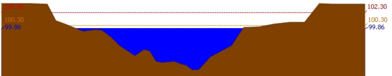
120112T แม่น้ำป่าสักที่บ้านหนองแหวน ต.วังมะข่อ อ.เมือง จ.เพชรบูรณ์ ระดับน้ำ 99.86 ม.รทก.
