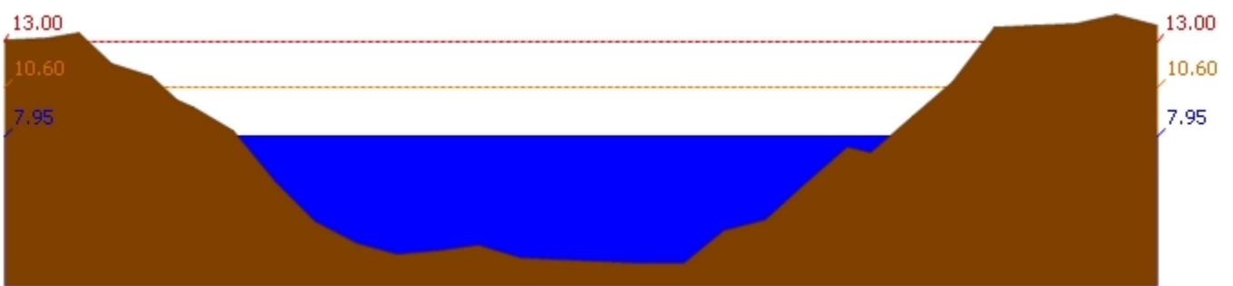
สถานี 120106T แม่น้ำป่าสักที่ อ.เสนาห์ ต.ศาลาวิไทย อ.เสนาห์ จ.สระบุรี ระดับน้ำ 7.95 ม.รทก.
