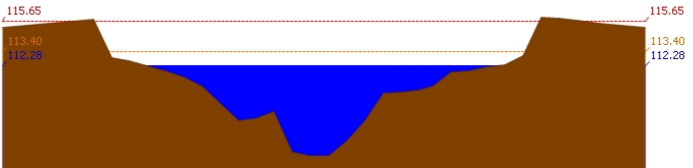
สถานี 120107T แม่น้ำป่าสักที่ อ.เมืองเพชรบูรณ์ ต.นาป่า อ.เมือง จ.เพชรบูรณ์ ระดับน้ำ 112.28 ม.รทก.
