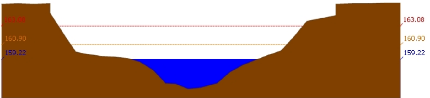
สถานี 120105T แม่น้ำป่าสักที่บ้านวังมเหนือ ต.ท่าอิบุญ อ.หล่มสัก จ.เพชรบูรณ์ ระดับน้ำ 159.22 ม.รทก.
