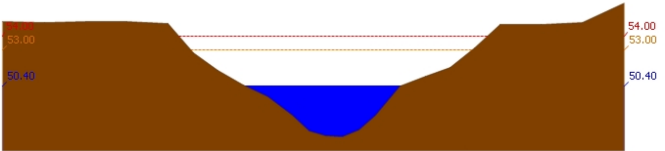
สถานี 120702T ลำสนธิที่บ้านท่าช้าง ต.หนองขาหย่าง อ.ชัยบาดาล จ.ลพบุรี ระดับน้ำ 50.40 ม.รทก.
