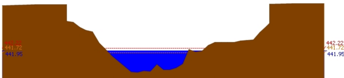
สถานี 060905T น้ำแม่ลี้ที่อำเภอลี้ ต.ลี้ อ.ลี้ จ.ลำพูน ระดับน้ำ 441.95 ม.รทก.
