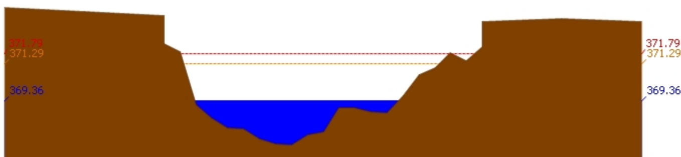
สถานี 060109T แม่น้ำปิงที่บ้านสบฮ้อย ต.แม่ระ อ.เชียงดาว จ.เชียงใหม่ ระดับน้ำ 369.36 ม.รทก.
