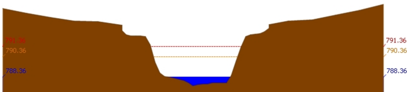
สถานี 061503T น้ำแม่ต้นที่บ้านคอย ต.ยางเปียง อ.อมก๋อย จ.เชียงใหม่ ระดับน้ำ 788.36 ม.รทก.
