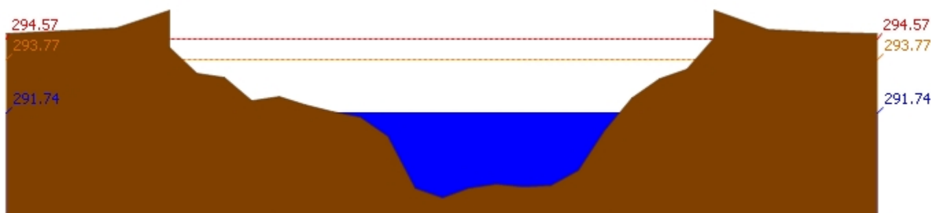
สถานี 060709T น้ำแม่กวังที่ลำพูน ต.เวียงของ อ.เมือง จ.ลำพูน ระดับน้ำ 291.74 ม.รทก.
