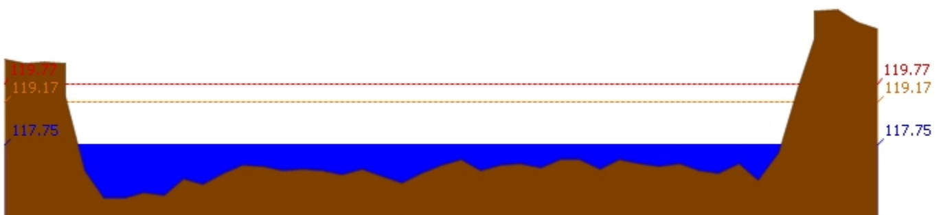
สถานี 060111T แม่น้ำปิงที่บ้านปากร่องห้วยจี้ ต.ตากออก อ.บ้านตาก จ.ตาก ระดับน้ำ 117.75 ม.รทก.
