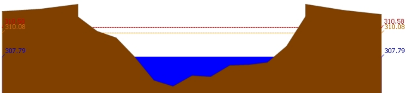
สถานี 060814T น้ำแม่ขานที่บ้านท่าโป่ง ต.บ้านแม่ อ.สันป่าตอง จ.เชียงใหม่ ระดับน้ำ 307.79 ม.รทก.
