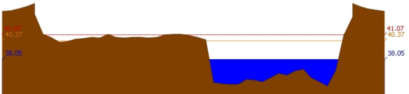
สถานี 060110T แม่น้ำปิงที่บ้านบางแก้ว ต.บางแก้ว อ.บรรพตพิสัย จ.นครสวรรค์ ระดับน้ำ 38.05 ม.รทก.
