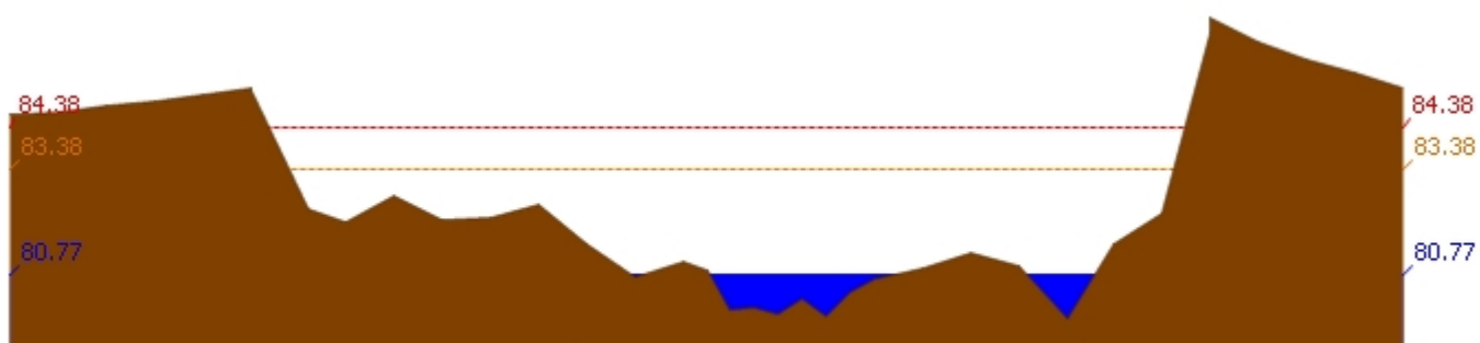
สถานี 062001T คลองสวนหมากที่บ้านน้ำไทรง ต.ท่าขุนราม อ.เมือง จ.กำแพงเพชร ระดับน้ำ 80.77 ม.รทก.
