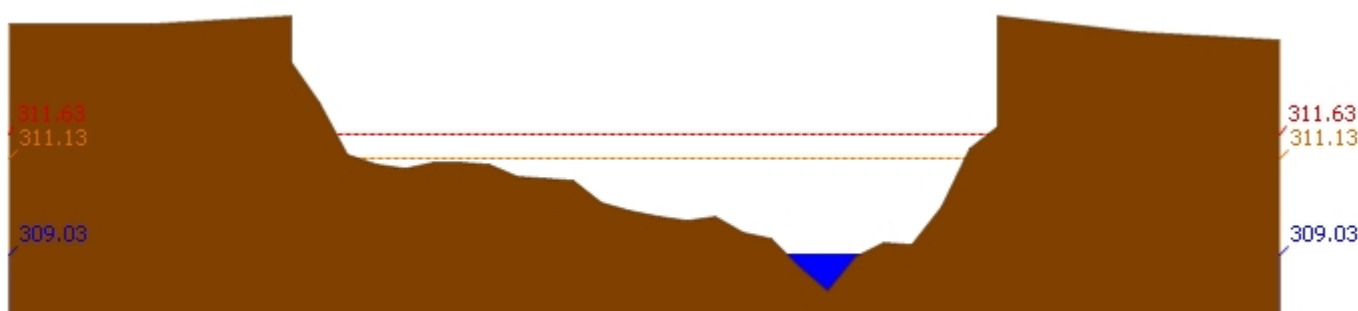
สถานี 061401T น้ำแม่หาดที่บ้านโป่งทุ่ง ต.โป่งทุ่ง อ.คอยเต่า จ.เชียงใหม่ ระดับน้ำ 309.03 ม.รทก.
