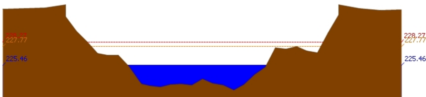
สถานี 070113T แม่น้ำวังที่ จ.ลำปาง ต.เวียงเหนือ อ.เมืองลำปาง จ.ลำปาง ระดับน้ำ 225.46 ม.รทก.
