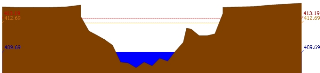
สถานี 070110T แม่น้ำวังที่ อ.วังเหนือ ต.วังเหนือ อ.วังเหนือ จ.ลำปาง ระดับน้ำ 409.69 ม.รทก.
