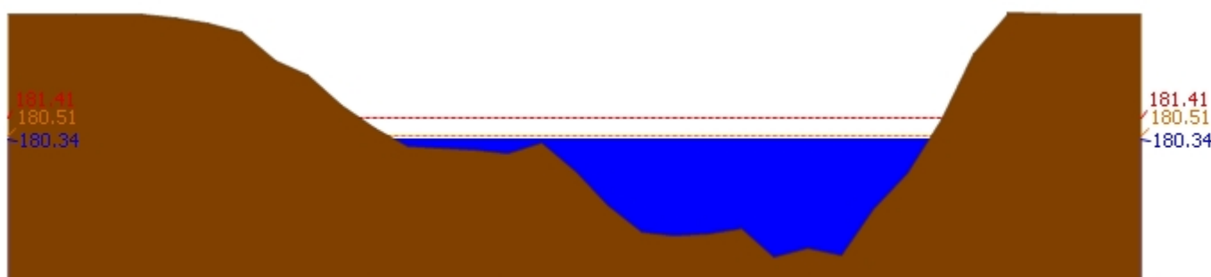
สถานี 070116T แม่น้ำวังที่บ้านแม่เตี๊ยะ ต.แม่ถอด อ.เถิน จ.ลำปาง ระดับน้ำ 180.34 ม.รทก.
