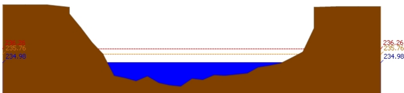
สถานี 070114T แม่น้ำวังที่บ้านปางชัย ต.บ้านเสด็จ อ.เมืองลำปาง จ.ลำปาง ระดับน้ำ 234.98 ม.รทก.
