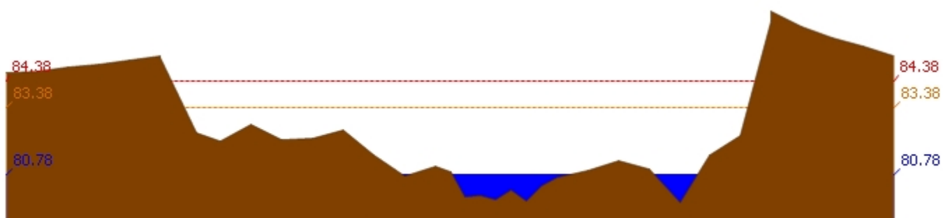
สถานี 062001T คลองสวนหมากที่บ้านน้ำไทรง ต.ท่าขุนราม อ.เมือง จ.กำแพงเพชร ระดับน้ำ 80.78 ม.รทก.
