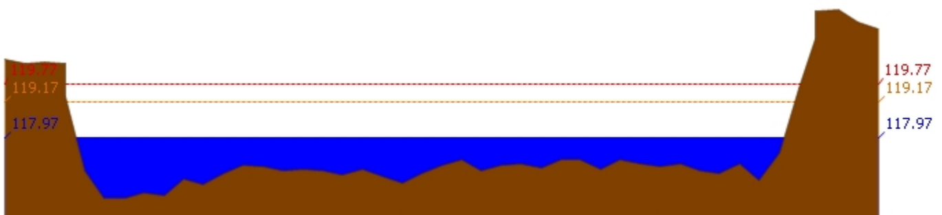
สถานี 060111T แม่น้ำปิงที่บ้านปากโรงห้วยจี้ ต.ตากออก อ.บ้านตาก จ.ตาก ระดับน้ำ 117.97 ม.รทก.
