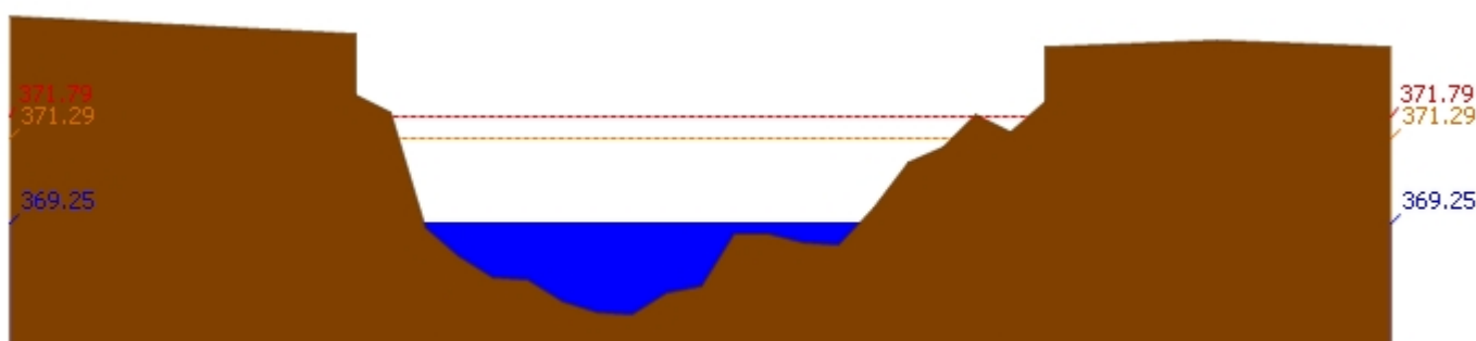
สถานี 060109T แม่น้ำปิงที่บ้านสบฮ้อย ต.แม่ระ อ.เชียงดาว จ.เชียงใหม่ ระดับน้ำ 369.25 ม.รทก.
