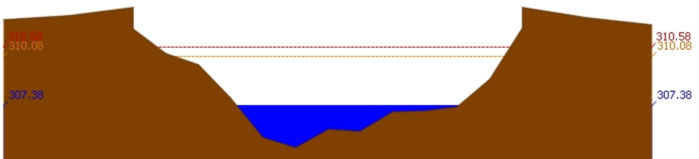
สถานี 060814T น้ำแม่ขานที่บ้านท่าโป่ง ต.บ้านแม่ อ.สันป่าตอง จ.เชียงใหม่ ระดับน้ำ 307.38 ม.รทก.
