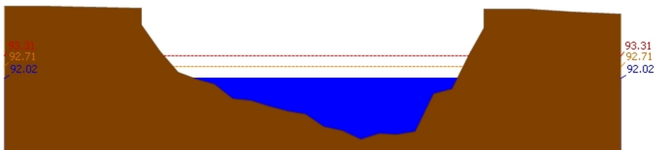
สถานี 061901T คลองแม่ระกาที่บ้านวังชะโอน ต.ท่าไม้ อ.พรานกระต่าย จ.กำแพงเพชร ระดับน้ำ 92.02 ม.รทก.
