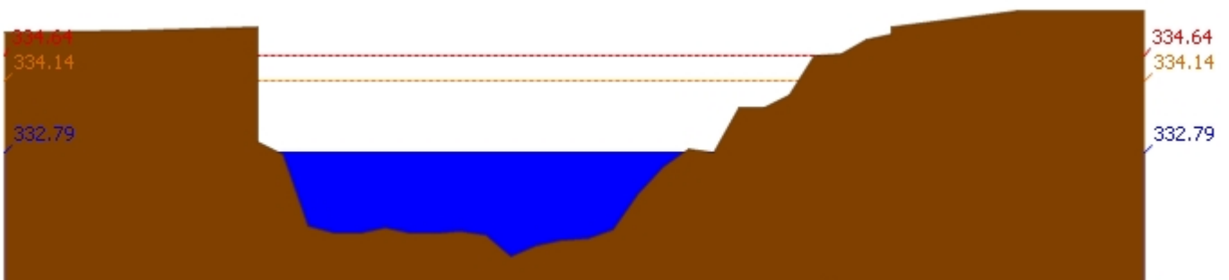
สถานี 070304T น้ำแม่สอยที่บ้านหนองกอก ต.แม่สุก อ.แจ้ห่ม จ.ลำปาง ระดับน้ำ 332.79 ม.รทก.
