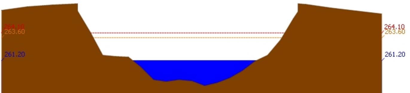
สถานี 070112T แม่น้ำวังที่บ้านบุญนาต ต.บุญนาตพัฒนา อ.เมืองลำปาง จ.ลำปาง ระดับน้ำ 261.20 ม.รทก.
