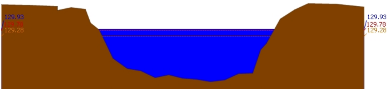
สถานี 070118T แม่น้ำวังที่บ้านแม่สลิด ต.แม่สลิด อ.บ้านตาก จ.ตาก ระดับน้ำ 129.93 ม.รทก.
