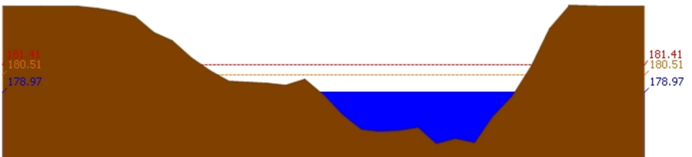
สถานี 070116T แม่น้ำวังที่บ้านแม่เตี๊ยะ ต.แม่ถอด อ.เถิน จ.ลำปาง ระดับน้ำ 178.97 ม.รทก.
