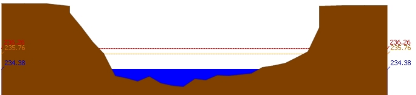
สถานี 070114T แม่น้ำวังที่บ้านปงชัย ต.บ้านเสด็จ อ.เมืองลำปาง จ.ลำปาง ระดับน้ำ 234.38 ม.รทก.
