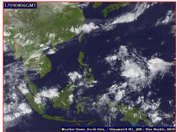
ภาพถ่ายจากดาวเทียม วันที่ ๘ ก.ย. ๒๕๖๐ เวลา ๑๓.๐๐ น.
