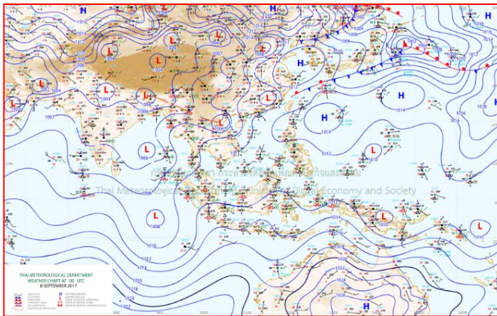
แผนที่อากาศ วันที่ ๘ ก.ย. ๒๕๖๐ เวลา ๐๗.๐๐ น.
