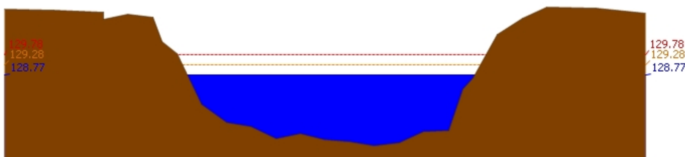
สถานี 070118T แม่น้ำวังที่บ้านแม่สลิด ต.แม่สลิด อ.บ้านตาก จ.ตาก ระดับน้ำ 128.77 ม.รทก.
