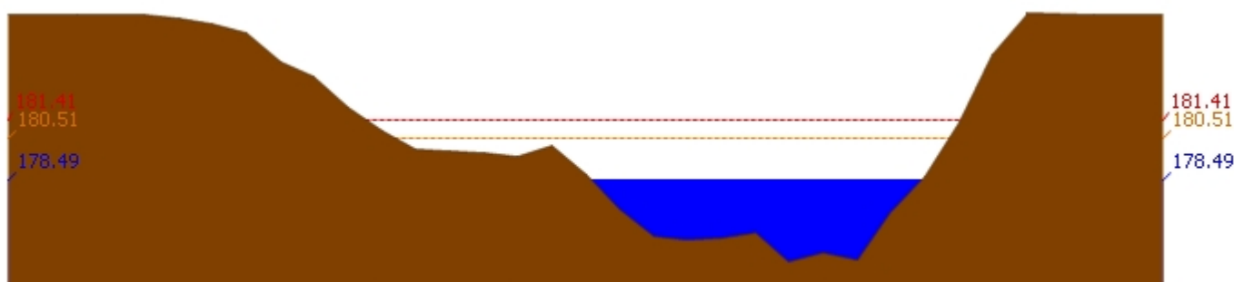
สถานี 070116T แม่น้ำวังที่บ้านแม่เตี๊ยะ ต.แม่ถอด อ.เถิน จ.ลำปาง ระดับน้ำ 178.49 ม.รทก.
