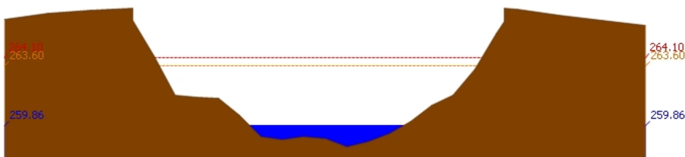
สถานี 070112T แม่น้ำวังที่บ้านบุญนาคร ต.บุญนาครพัฒนา อ.เมืองลำปาง จ.ลำปาง ระดับน้ำ 259.86 ม.รทก.
