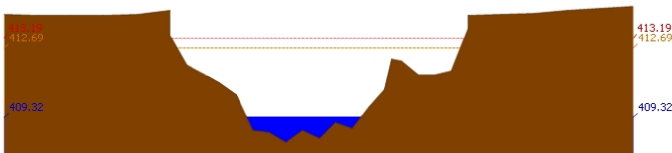
สถานี 070110T แม่น้ำวังที่ อ.วังเหนือ ต.วังเหนือ อ.วังเหนือ จ.ลำปาง ระดับน้ำ 409.32 ม.รทก.
