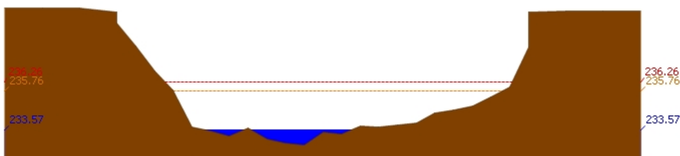
สถานี 070114T แม่น้ำวังที่บ้านปงชัย ต.บ้านเสด็จ อ.เมืองลำปาง จ.ลำปาง ระดับน้ำ 233.57 ม.รทก.
