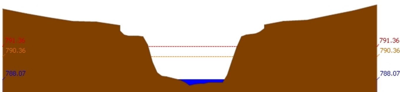
สถานี 061503T น้ำแม่ต้นที่บ้านคอย ต.ยางเปียง อ.อมก๋อย จ.เชียงใหม่ ระดับน้ำ 788.07 ม.รทก.
