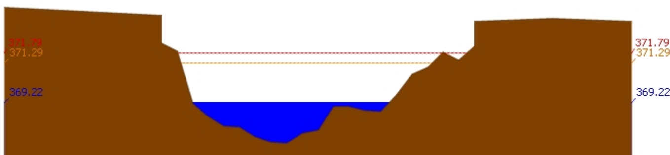
สถานี 060109T แม่น้ำปิงที่บ้านสบอ้อ ต.แม่ปะ อ.เชียงดาว จ.เชียงใหม่ ระดับน้ำ 369.22 ม.รทก.
