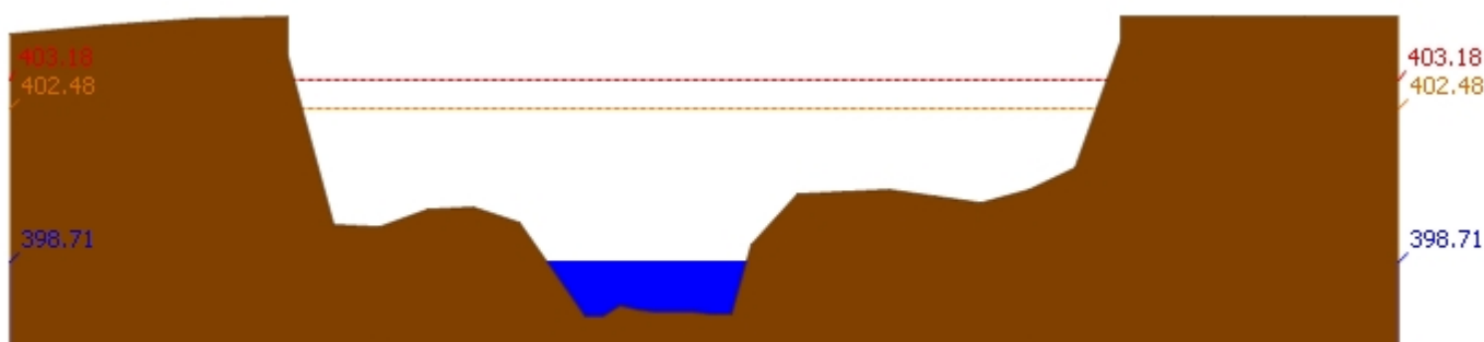
สถานี 060305T น้ำแม่จืดที่บ้านโป่งบัวบาน ต.แม่ป๋อง อ.พร้าว จ.เชียงใหม่ ระดับน้ำ 398.71 ม.รทก.
