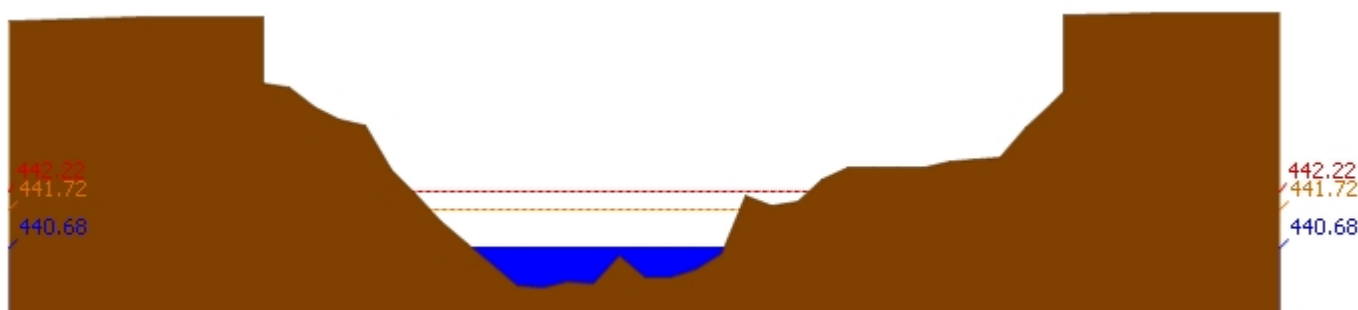
สถานี 060905T น้ำแม่ลี้ที่อำเภอลี้ ต.ลี้ อ.ลี้ จ.ลำพูน ระดับน้ำ 440.68 ม.รทก.
