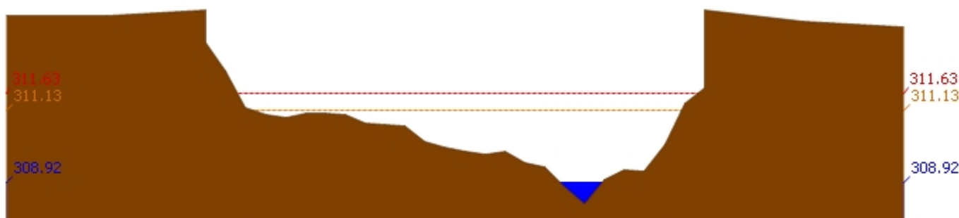
สถานี 061401T น้ำแม่หาดที่บ้านโป่งทุ่ง ต.โป่งทุ่ง อ.คอยเต่า จ.เชียงใหม่ ระดับน้ำ 308.92 ม.รทก.
