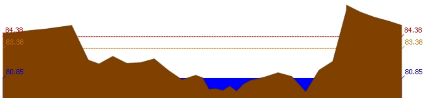
สถานี 062001T คลองสวนหมากที่บ้านน้ำไทรง ต.ท่าขุนราม อ.เมือง จ.กำแพงเพชร ระดับน้ำ 80.85 ม.รทก.
