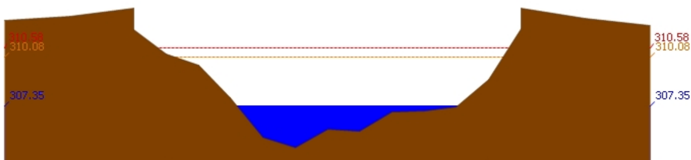
สถานี 060814T น้ำแม่ขานที่บ้านท่าโป่ง ต.บ้านแม อ.สันป่าตอง จ.เชียงใหม่ ระดับน้ำ 307.35 ม.รทก.
