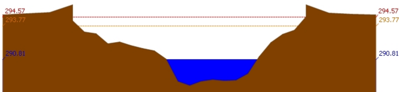
สถานี 060709T น้ำแม่กวงที่ลำพูน ต.เวียงยอง อ.เมือง จ.ลำพูน ระดับน้ำ 290.81 ม.รทก.
