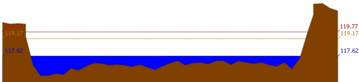
สถานี 060111T แม่น้ำปิงที่บ้านปากร่องห้วยจี้ ต.ตากออก อ.บ้านตาก จ.ตาก ระดับน้ำ 117.62 ม.รทก.
