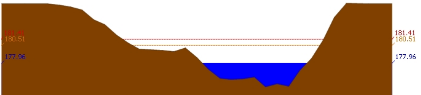
สถานี 070116T แม่น้ำวังที่บ้านแม่เตี๊ยะ ต.แม่ถอด อ.เถิน จ.ลำปาง ระดับน้ำ 177.96 ม.รทก.
