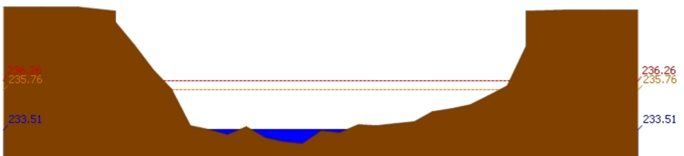
สถานี 070114T แม่น้ำวังที่บ้านปงชัย ต.บ้านเสด็จ อ.เมืองลำปาง จ.ลำปาง ระดับน้ำ 233.51 ม.รทก.
