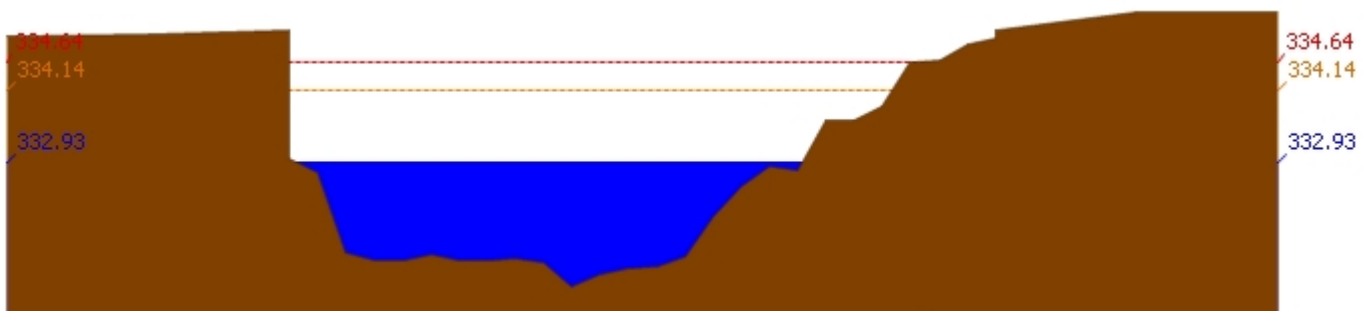
สถานี 070304T น้ำแม่สอยที่บ้านหนองกอก ต.แม่สุก อ.แจ้ห่ม จ.ลำปาง ระดับน้ำ 332.93 ม.รทก.
