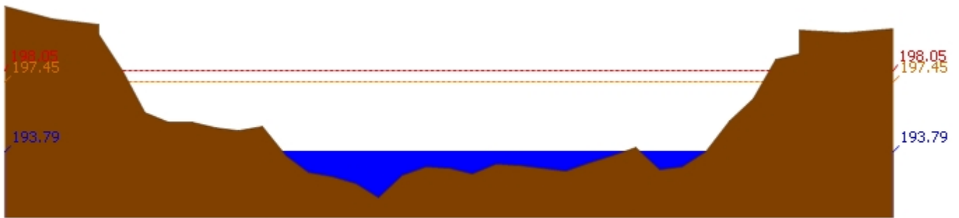
สถานี 070115T น้ำแม่วังที่บ้านอ้อ ต.แม่กัวะ อ.สบปราบ จ.ลำปาง ระดับน้ำ 193.79 ม.รทก.
