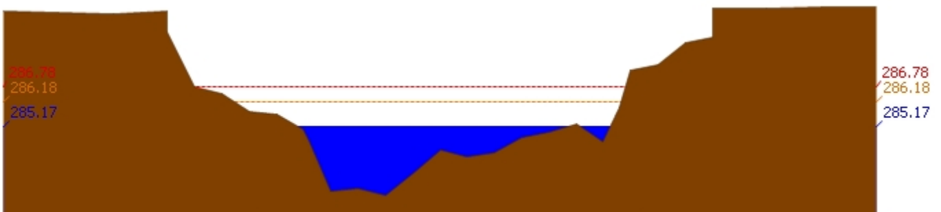
สถานี 070111T แม่น้ำวังที่บ้านแปงโปงชัย ต.บ้านเสา อ.แจ้ห่ม จ.ลำปาง ระดับน้ำ 285.17 ม.รทก.
