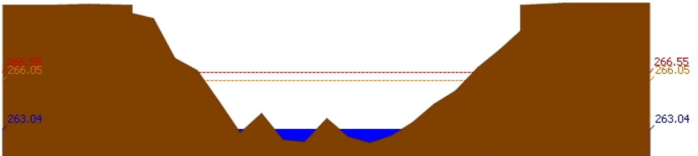
สถานี 070604T น้ำแม่จางที่บ้านสุโหมไชยมงคล ต.หัวเสือ อ.แม่ทะ จ.ลำปาง ระดับน้ำ 263.04 ม.รทก.
