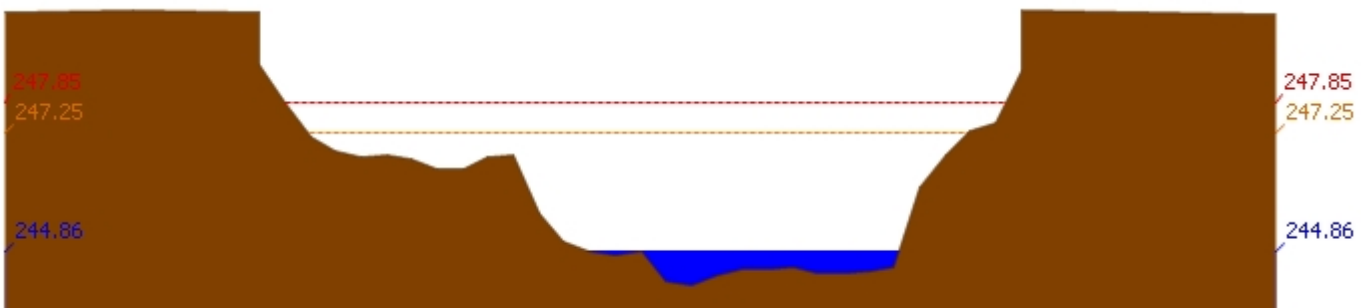
สถานี 070403T น้ำแม่คู่ยที่บ้านแค้ ต.บ้านเป้า อ.เมืองลำปาง จ.ลำปาง ระดับน้ำ 244.86 ม.รทก.
