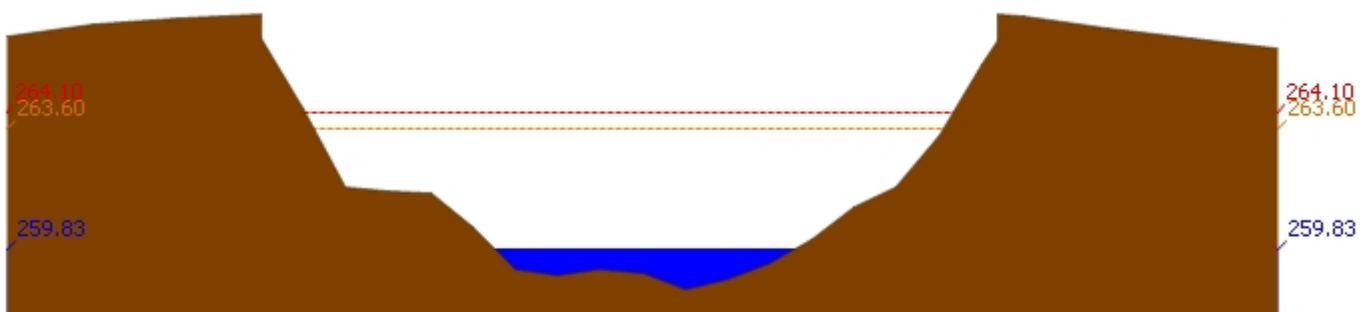
สถานี 070112T แม่น้ำวังที่บ้านบุญนาต ต.บุญนาตพัฒนา อ.เมืองลำปาง จ.ลำปาง ระดับน้ำ 259.83 ม.รทก.
