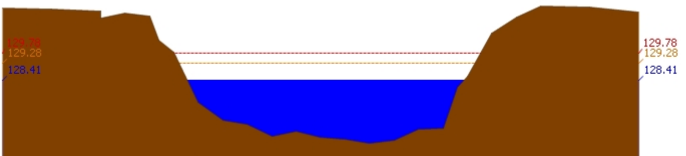
สถานี 070118T แม่น้ำวังที่บ้านแม่สลิด ต.แม่สลิด อ.บ้านตาก จ.ตาก ระดับน้ำ 128.41 ม.รทก.
