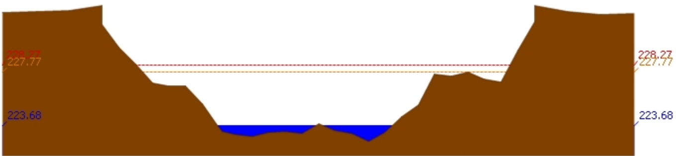
สถานี 070113T แม่น้ำวังที่ จ.ลำปาง ต.เวียงเหนือ อ.เมืองลำปาง จ.ลำปาง ระดับน้ำ 223.68 ม.รทก.
