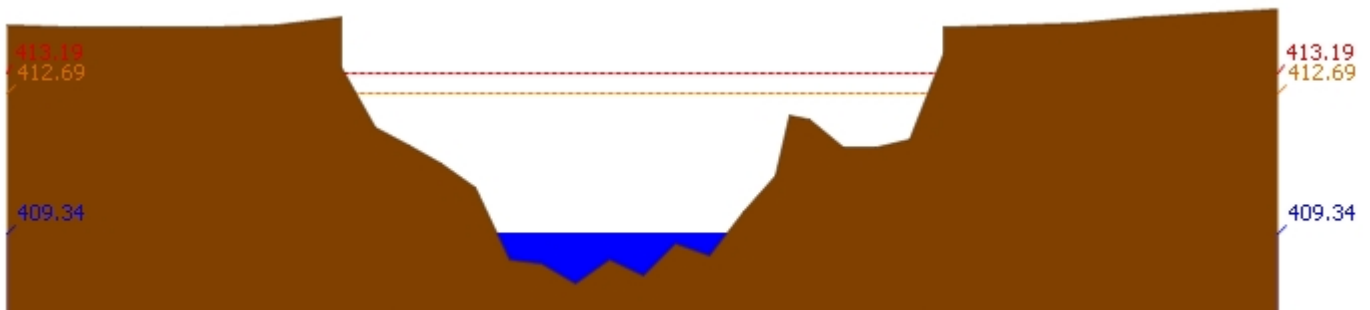
สถานี 070110T แม่น้ำวังที่ อ.วังเหนือ ต.วังเหนือ อ.วังเหนือ จ.ลำปาง ระดับน้ำ 409.34 ม.รทก.
