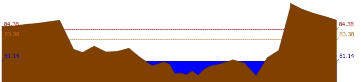
สถานี 062001T คลองสวนหมากที่บ้านน้ำไทรง ต.ท่าขุนราม อ.เมือง จ.กำแพงเพชร ระดับน้ำ 81.14 ม.รทก.
