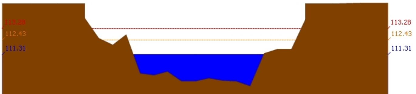
สถานี 061801T คลองวังเจ้าที่บ้านคลองลึก ต.เชียงทอง อ.วังเจ้า จ.ตาก ระดับน้ำ 111.31 ม.รทก.
