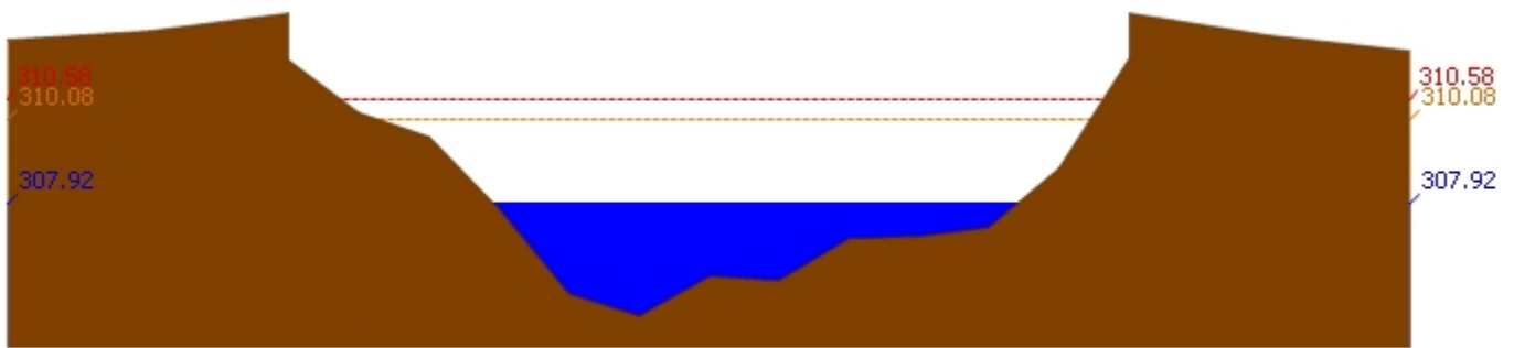
สถานี 060814T น้ำแม่ขานที่บ้านท่าโป่ง ต.บ้านแม่ อ.สันป่าตอง จ.เชียงใหม่ ระดับน้ำ 307.92 ม.รทก.
