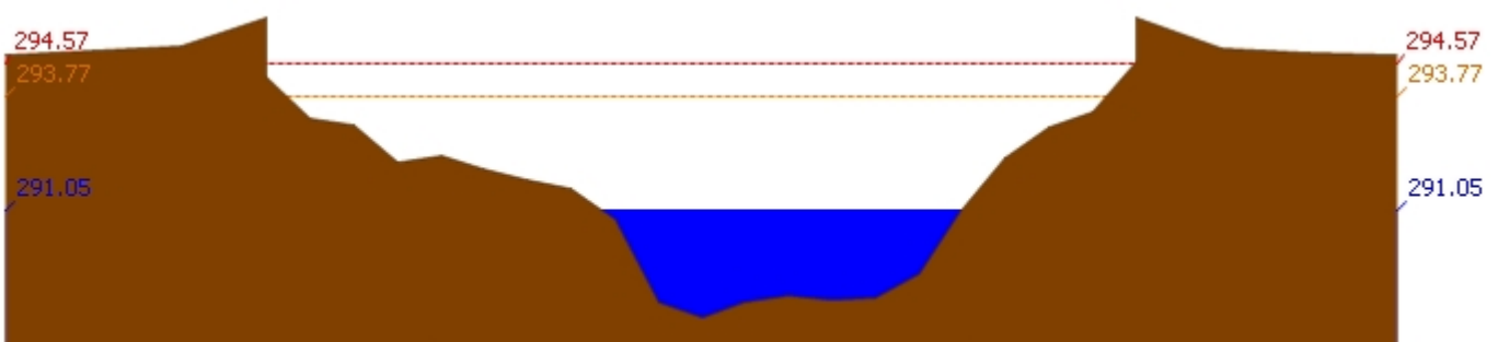
สถานี 060709T น้ำแม่กวงที่ลำพูน ต.เวียงยอง อ.เมือง จ.ลำพูน ระดับน้ำ 291.05 ม.รทก.
