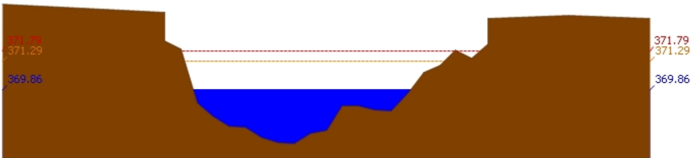
สถานี 060109T แม่น้ำปิงที่บ้านสบอ้อ ต.แม่ปะ อ.เชียงดาว จ.เชียงใหม่ ระดับน้ำ 369.86 ม.รทก.
