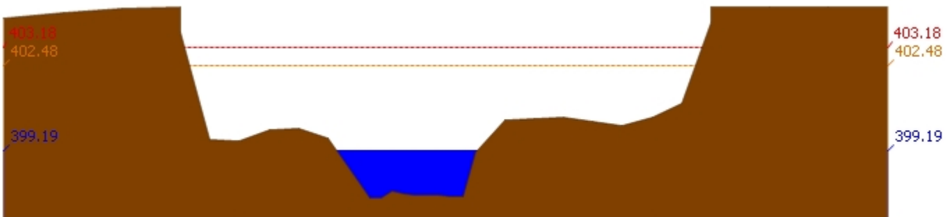
สถานี 060305T น้ำแม่จืดที่บ้านโป่งบัวบาน ต.แม่ป๋อง อ.พร้าว จ.เชียงใหม่ ระดับน้ำ 399.19 ม.รทก.
