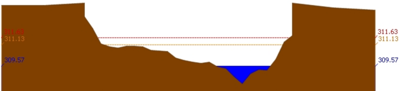
สถานี 061401T น้ำแม่หาดที่บ้านโป่งทุ่ง ต.โป่งทุ่ง อ.คอยเต่า จ.เชียงใหม่ ระดับน้ำ 309.57 ม.รทก.
