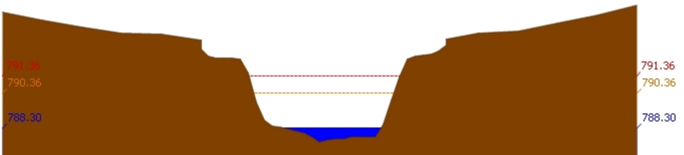
สถานี 061503T น้ำแม่ต้นที่บ้านคอย ต.ยางเปียง อ.อมก๋อย จ.เชียงใหม่ ระดับน้ำ 788.30 ม.รทก.
