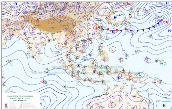
แผนที่อากาศ วันที่ ๒๕ ก.ย. ๒๕๖๐ เวลา ๐๑.๐๐ น.
