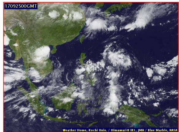
ภาพถ่ายจากดาวเทียม วันที่ ๒๕ ก.ย. ๒๕๖๐ เวลา ๐๗.๐๐ น.
