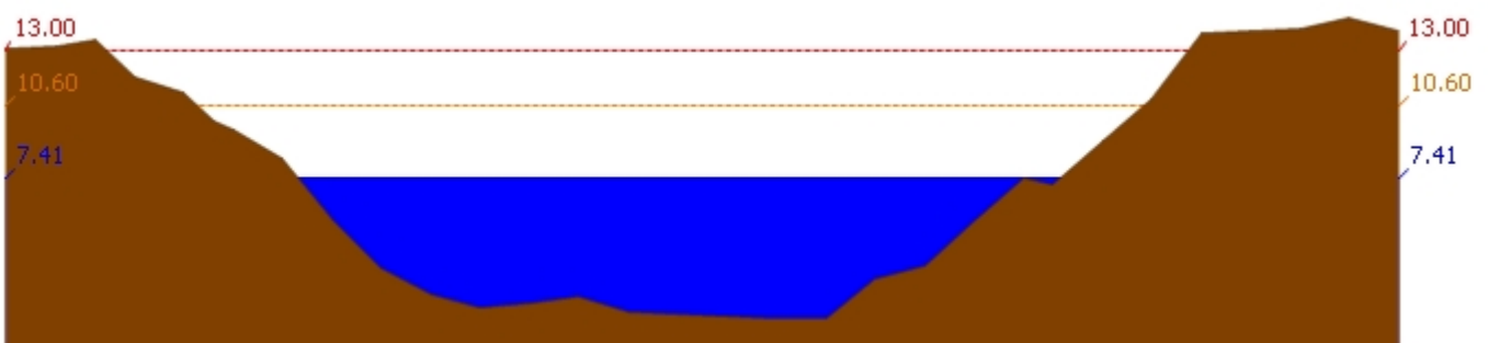
สถานี 120106T แม่น้ำป่าสักที่ อ.เสนาห์ ต.ศาลาวิไทย อ.เสนาห์ จ.สระบุรี ระดับน้ำ 7.41 ม.รทก.
