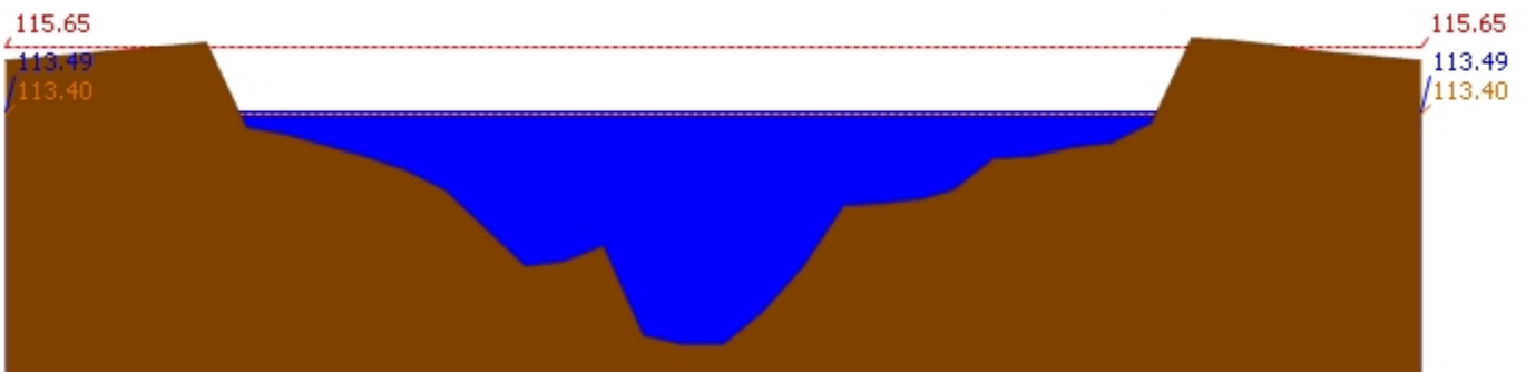
สถานี 120107T แม่น้ำป่าสักที่ อ.เมืองเพชรบูรณ์ ต.นาป่า อ.เมือง จ.เพชรบูรณ์ ระดับน้ำ 113.49 ม.รทก.
