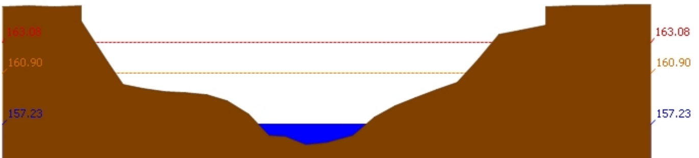
สถานี 120105T แม่น้ำป่าสักที่บ้านวังมเหนือก ต.ท่าอิบุญ อ.หล่มสัก จ.เพชรบูรณ์ ระดับน้ำ 157.23 ม.รทก.
