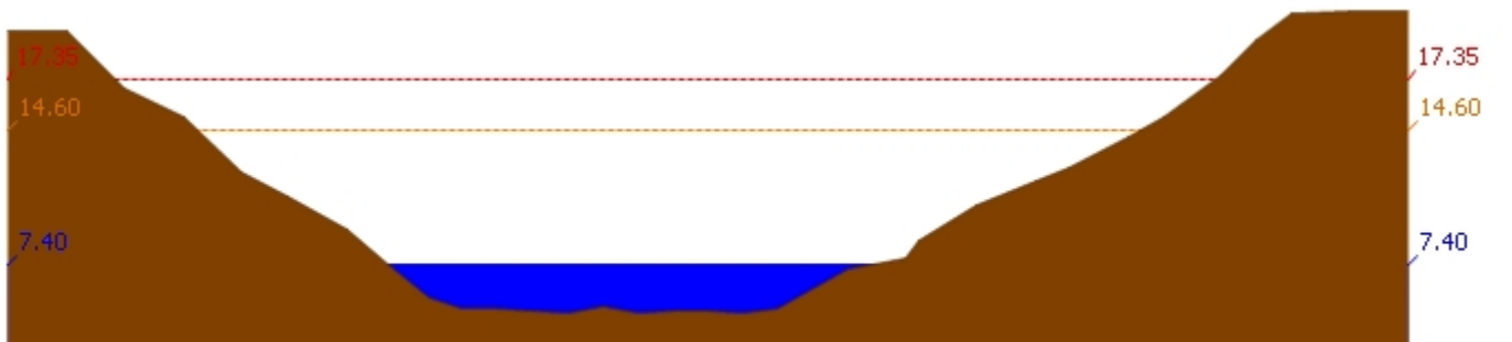
สถานี 120109T แม่น้ำป่าสักที่ อ.แก่งคอย ต.แก่งคอย อ.แก่งคอย จ.สระบุรี ระดับน้ำ 7.40 ม.รทก.
