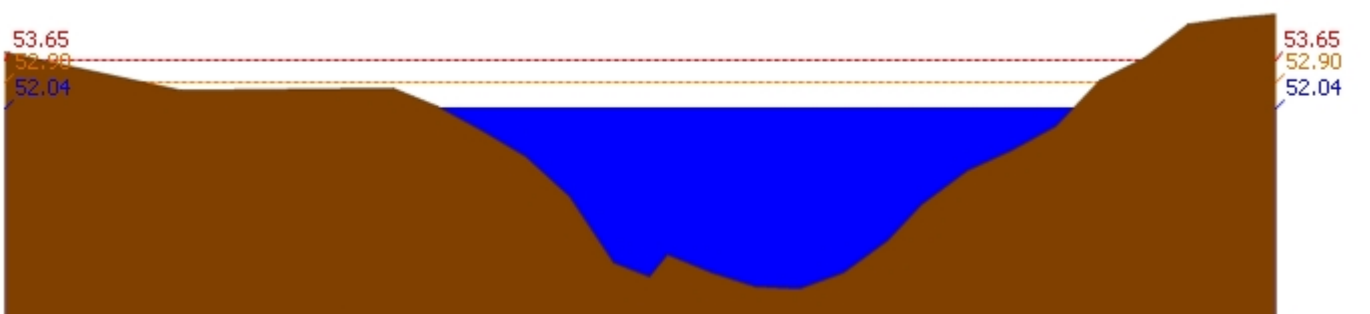
สถานี 120113T แม่น้ำป่าสักที่บ้านเขาค้าง ต.คลองกระจิง อ.ศรีเทพ จ.เพชรบูรณ์ ระดับน้ำ 52.04 ม.รทก.
