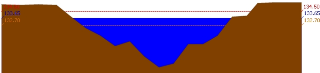
สถานี 120111T แม่น้ำป่าสักที่บ้านจางวาง ต.ลานบัว อ.หล่มสัก จ.เพชรบูรณ์ ระดับน้ำ 133.65 ม.รทก.
