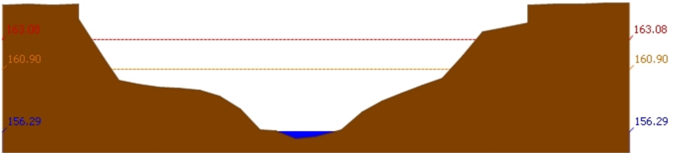
สถานี 120105T แม่น้ำป่าสักที่บ้านวังมเสหนือ ต.ทำอัญญ อ.หล่มสัก จ.เพชรบูรณ์ ระดับน้ำ 156.29 ม.รทก.
