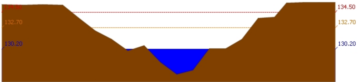
สถานี 120111T แม่น้ำป่าสักที่บ้านจางวาง ต.ลานบัว อ.หล่มสัก จ.เพชรบูรณ์ ระดับน้ำ 130.20 ม.รทก.
