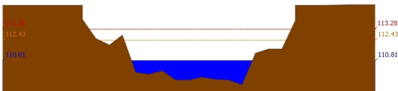
สถานี 061801T คลองวังเจ้าที่บ้านคลองลึก ต.เชียงทอง อ.วังเจ้า จ.ตาก ระดับน้ำ 110.81 ม.รทก.
