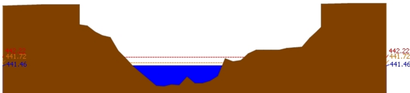
สถานี 060905T น้ำแม่ลี้ที่อำเภอเถิน ต.ลี้ อ.ลี้ จ.ลำพูน ระดับน้ำ 441.46 ม.รทก.
