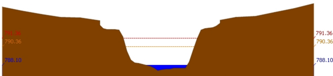
สถานี 061503T น้ำแม่ต้นที่บ้านคอย ต.ยางเปียง อ.อมก๋อย จ.เชียงใหม่ ระดับน้ำ 788.10 ม.รทก.
