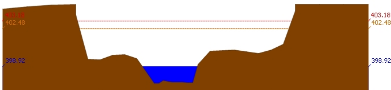
สถานี 060305T น้ำแม่จัดที่บ้านโป่งบัวบาน ต.แม่ป๋อง อ.พร้าว จ.เชียงใหม่ ระดับน้ำ 398.92 ม.รทก.
