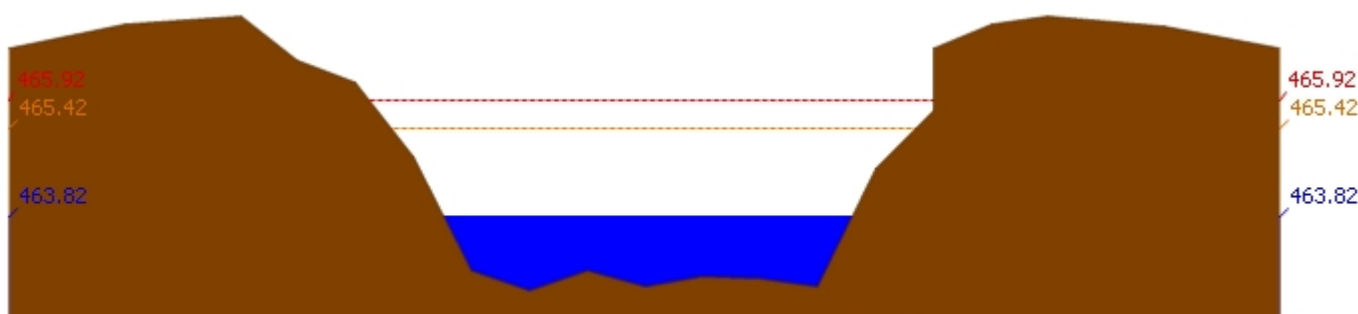
สถานี 061206T น้ำแม่แจ่มที่บ้านทัพ ต.ท่าผา อ.แม่แจ่ม จ.เชียงใหม่ ระดับน้ำ 463.82 ม.รทก.
