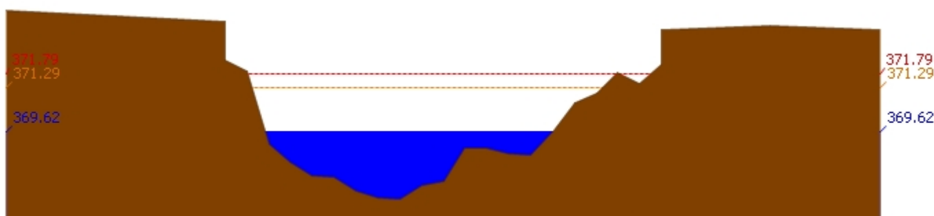
สถานี 060109T แม่น้ำปิงที่บ้านสบอ้อ ต.แม่ปะ อ.เชียงดาว จ.เชียงใหม่ ระดับน้ำ 369.62 ม.รทก.
