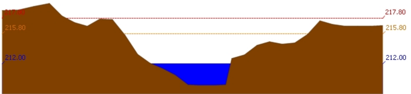
สถานี 120205T แม่น้ำป่าสักที่บ้านอู่กะทาด ต.ศิลา อ.หล่มเก่า จ.เพชรบูรณ์ ระดับน้ำ 212.00 ม.รทก.
