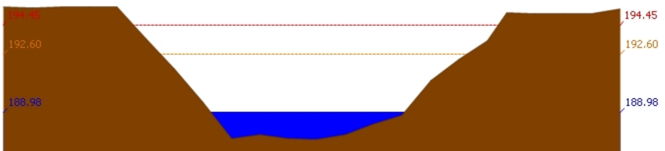
สถานี 120901T ห้วยมวกเหล็กที่ อ.มวกเหล็ก ต.มวกเหล็ก อ.มวกเหล็ก จ.สระบุรี ระดับน้ำ 188.98 ม.รทก.
