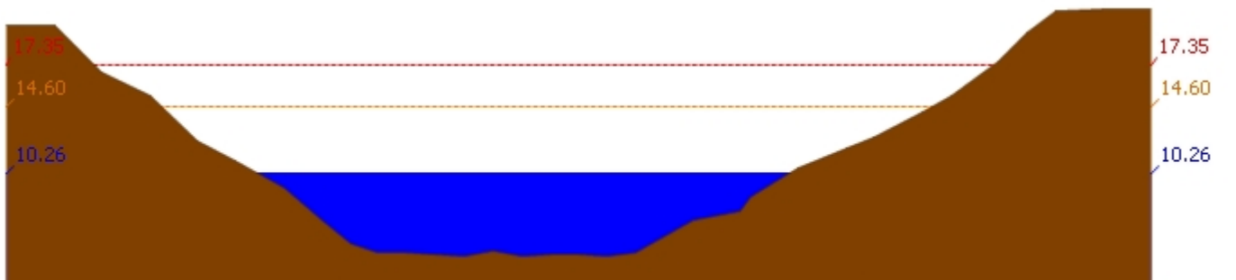
สถานี 120109T แม่น้ำป่าสักที่ อ.แก่งคอย ต.แก่งคอย อ.แก่งคอย จ.สระบุรี ระดับน้ำ 10.26 ม.รทก.
