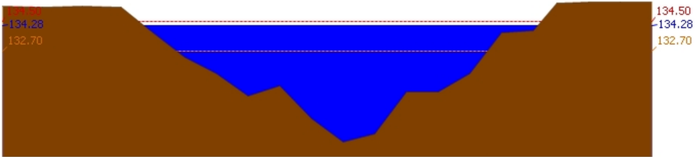
สถานี 120111T แม่น้ำป่าสักที่บ้านจางวาง ต.ลานบัว อ.หล่มสัก จ.เพชรบูรณ์ ระดับน้ำ 134.28 ม.รทก.
