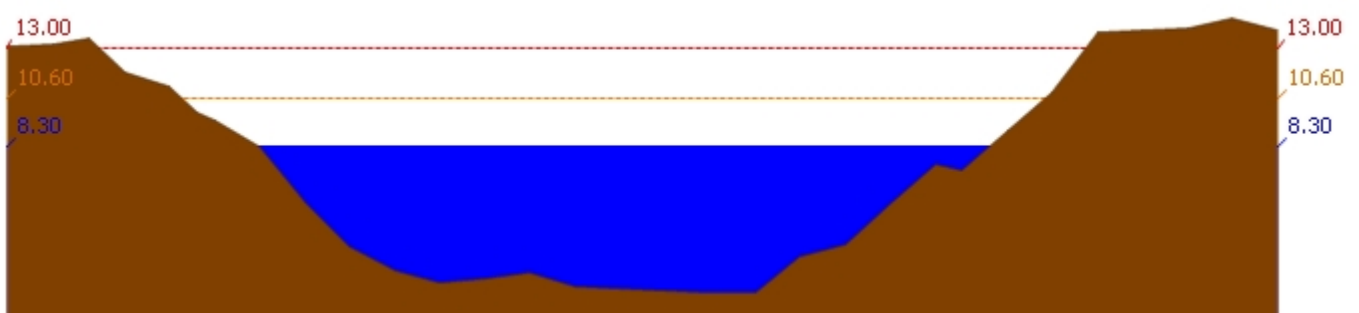
สถานี 120106T แม่น้ำป่าสักที่ อ.เสนาห์ ต.ศาลาวิไทย อ.เสนาห์ จ.สระบุรี ระดับน้ำ 8.30 ม.รทก.
