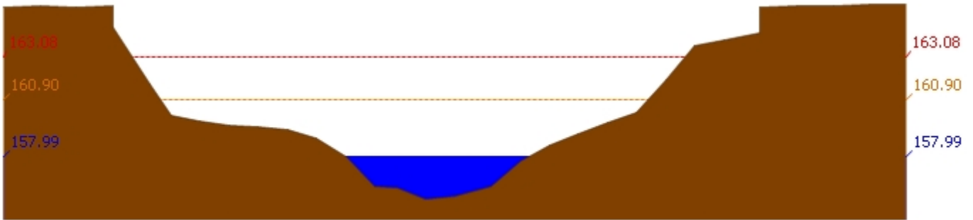
สถานี 120105T แม่น้ำป่าสักที่บ้านวังมเสหนือ ต.ท่าอิบุญ อ.หล่มสัก จ.เพชรบูรณ์ ระดับน้ำ 157.99 ม.รทก.
