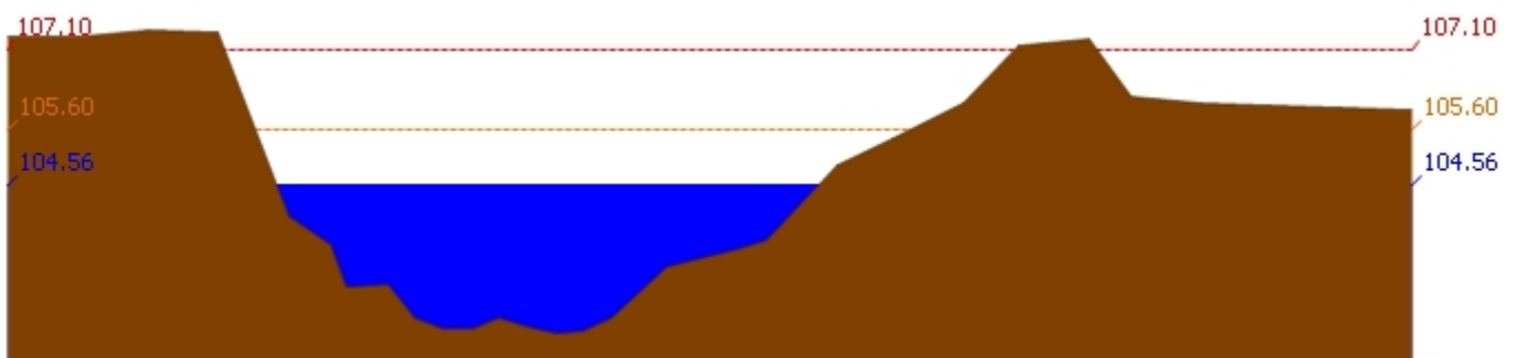
สถานี 110402T หัวขั้วทึบเสลาที่บ้านนาไร่เดียว ต.ลานสัก อ.ลานสัก จ.อุทัยธานี ระดับน้ำ 104.56 ม.รทก.
