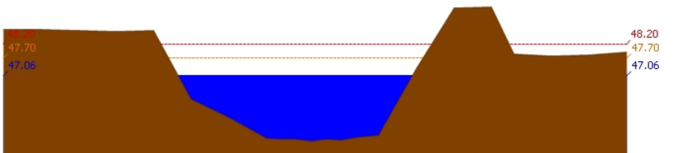
สถานี 110303T คลองโพธิ์ที่บ้านทุ่งสงบ ต.ไม้เขี้ยว อ.สว่างอารมณ์ จ.อุทัยธานี ระดับน้ำ 47.06 ม.รทก.
