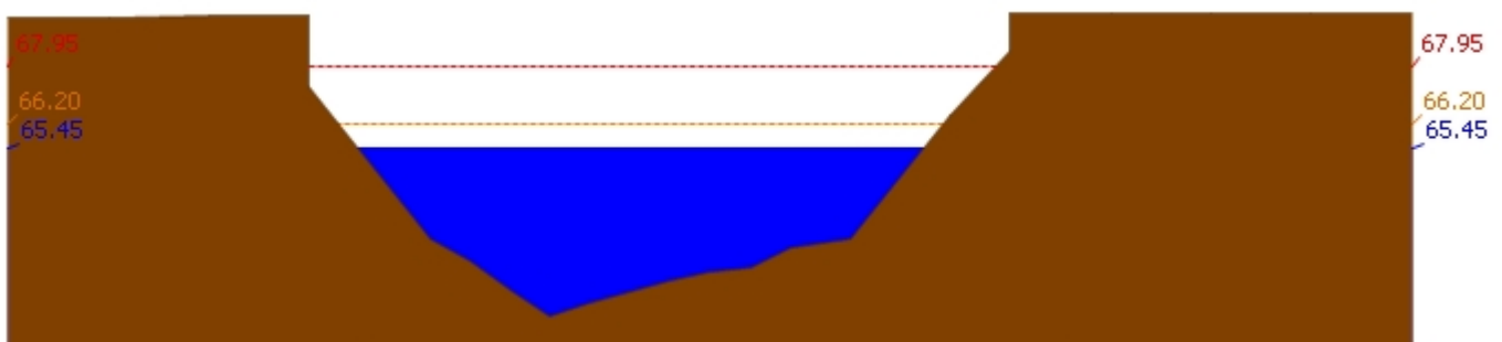
สถานี 110501T น้ำแมวกักที่บ้านคลองสาลี ต.ลาดยาว อ.ลาดยาว จ.นครสวรรค์ ระดับน้ำ 65.45 ม.รทก.
