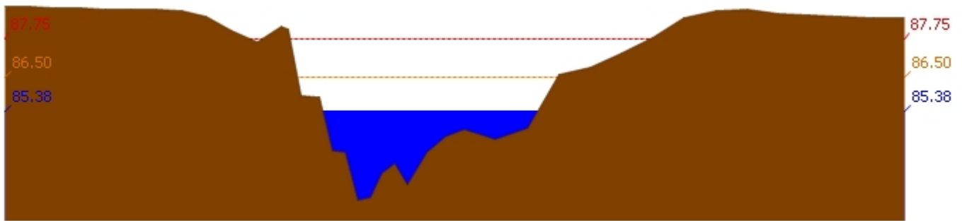
สถานี 110403T หัวขั้วตบเสลาที่บ้านดินแดง ต.ประตู่หิน อ.ลานสัก จ.อุทัยธานี ระดับน้ำ 85.38 ม.รทก.
