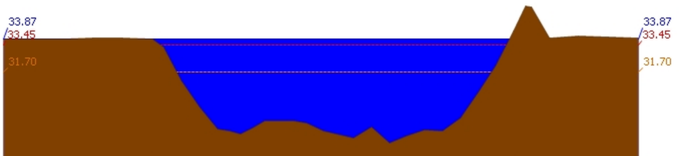
สถานี 110503T แม่น้ำตากแดดที่บ้านหนองขาลาย ต.หนองหลวง อ.สว่างอารมณ์ จ.อุทัยธานี ระดับน้ำ 33.87 ม.รทก.
