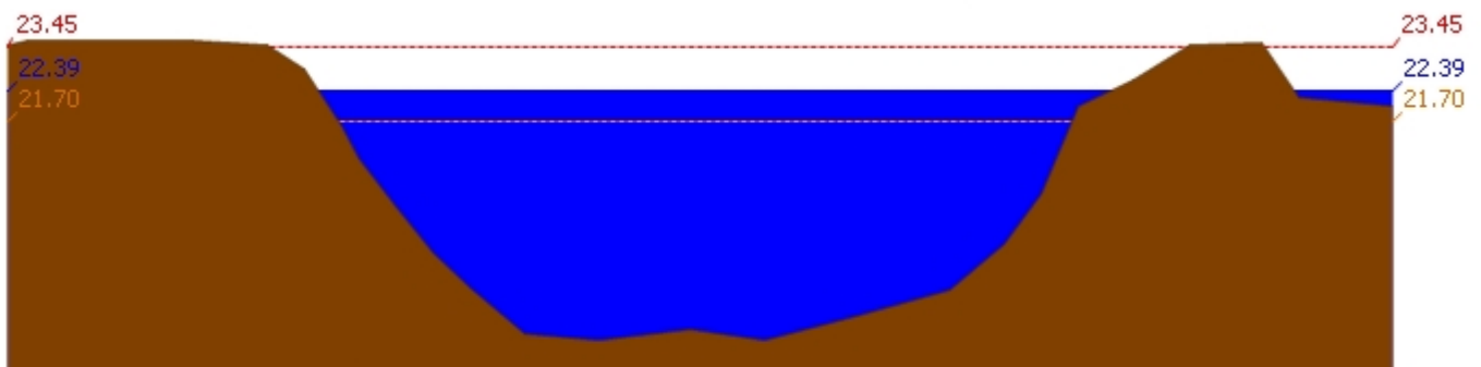
สถานี 110504T แม่น้ำตากแดดที่บ้านบุญลือ ต.เนินแจง อ.เมืองอุทัยธานี จ.อุทัยธานี ระดับน้ำ 22.39 ม.รทก.
