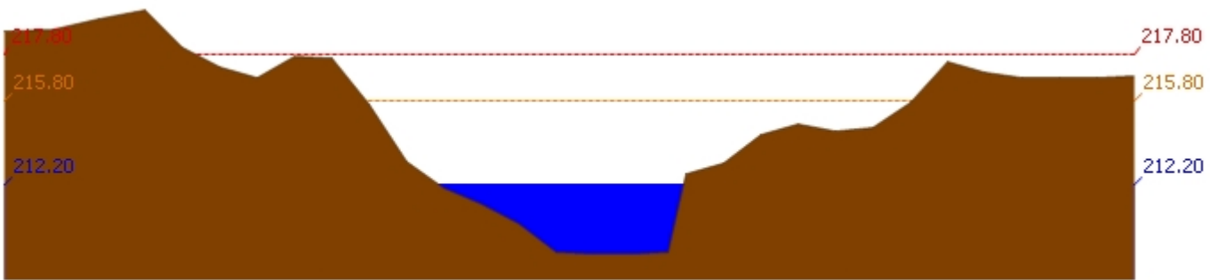
สถานี 120205T แม่น้ำป่าสักที่บ้านอู่กะทาด ต.ศิลา อ.หล่มเก่า จ.เพชรบูรณ์ ระดับน้ำ 212.20 ม.รทก.
