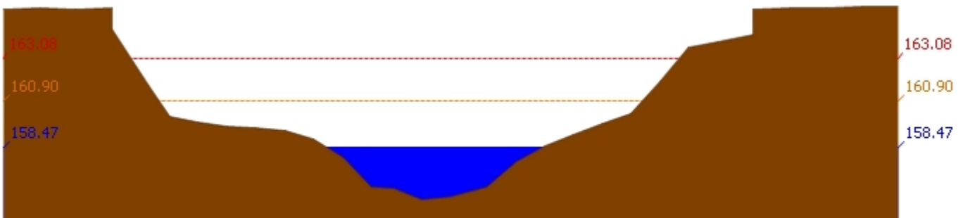
สถานี 120105T แม่น้ำป่าสักที่บ้านวังมเสหนือ ต.ทำอัญญ อ.หล่มสัก จ.เพชรบูรณ์ ระดับน้ำ 158.47 ม.รทก.
