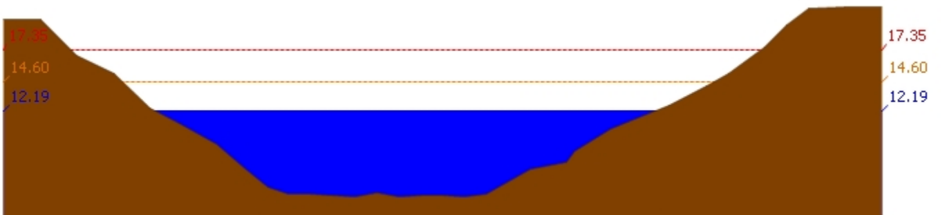
สถานี 120109T แม่น้ำป่าสักที่ อ.แก่งคอย ต.แก่งคอย อ.แก่งคอย จ.สระบุรี ระดับน้ำ 12.19 ม.รทก.
