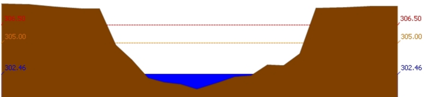
สถานี 120304T ห้วยน้ำพุที่บ้านกกกะบาก ต.โป่ง อ.ด่านซ้าย จ.เลย ระดับน้ำ 302.46 ม.รทก.
