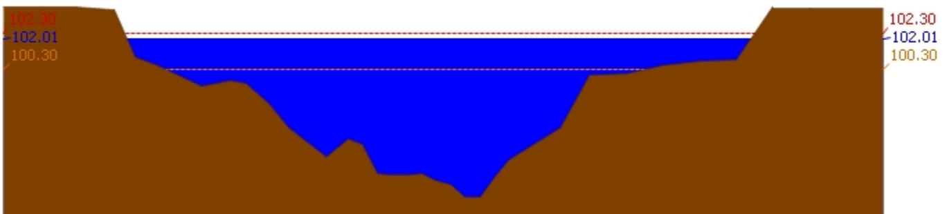
สถานี 120112T แม่น้ำป่าสักที่บ้านหนองแหวน ต.วังมะข่อ อ.เมือง จ.เพชรบูรณ์ ระดับน้ำ 102.01 ม.รทก.
