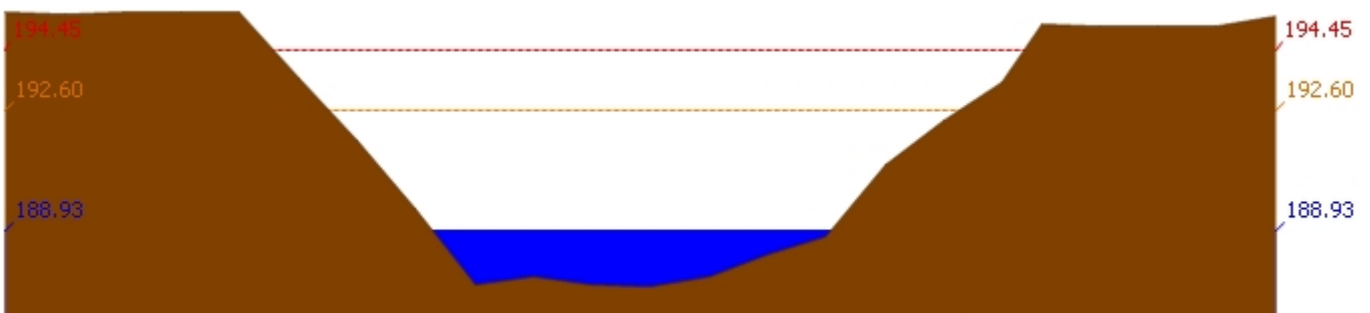
สถานี 120901T ห้วยมวกเหล็กที่ อ.มวกเหล็ก ต.มวกเหล็ก อ.มวกเหล็ก จ.สระบุรี ระดับน้ำ 188.93 ม.รทก.
