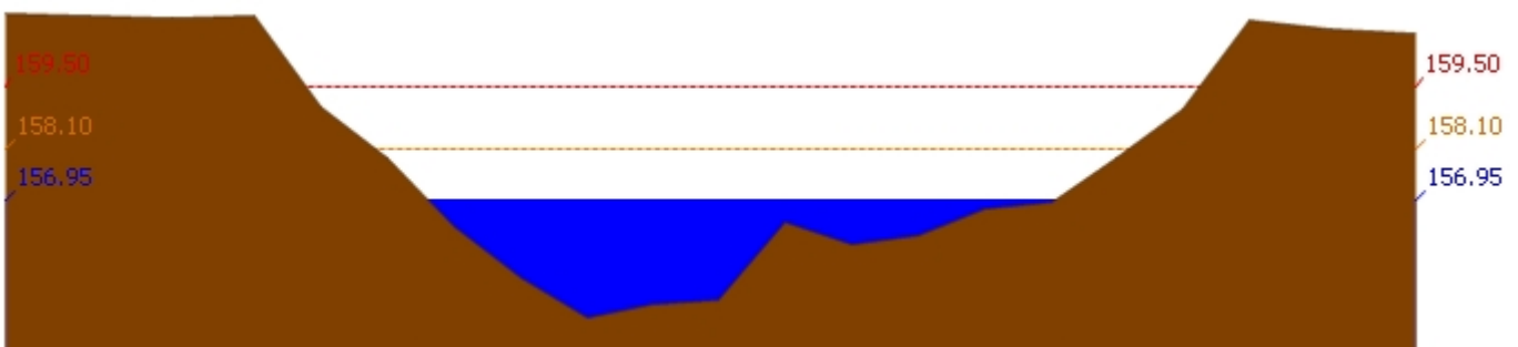
สถานี 120305T หัวน้ำพุที่ อ.หล่มเก่า ต.หล่มเก่า อ.หล่มเก่า จ.เพชรบูรณ์ ระดับน้ำ 156.95 ม.รทก.
