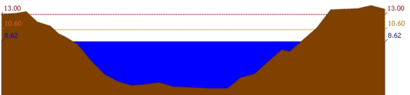
สถานี 120106T แม่น้ำป่าสักที่ อ.เสนาให้ ต.ศาลาวิไทย อ.เสนาให้ จ.สระบุรี ระดับน้ำ 8.62 ม.รทก.
