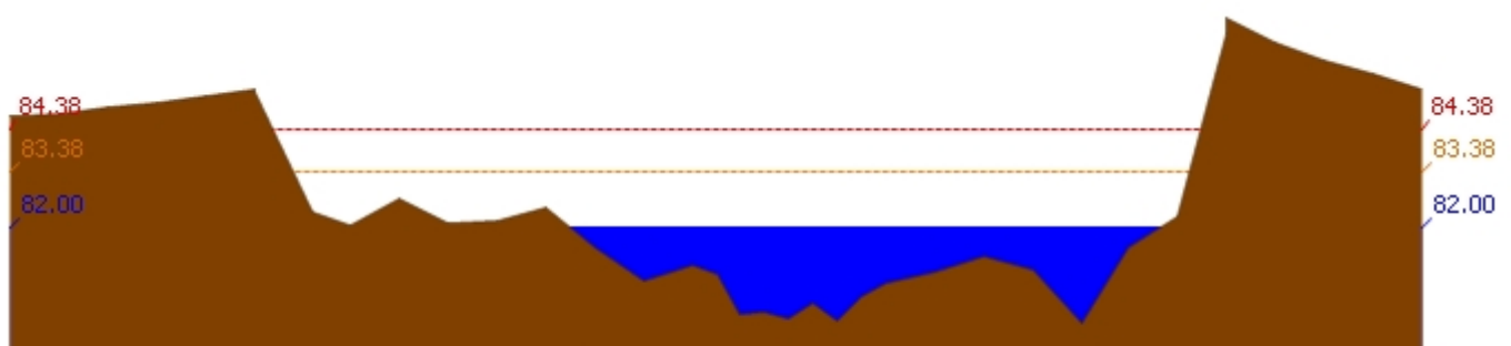
สถานี 062001T คลองสวนหมากที่บ้านน้ำไทรง ต.ท่าขุนราม อ.เมือง จ.กำแพงเพชร ระดับน้ำ 82.00 ม.รทก.
