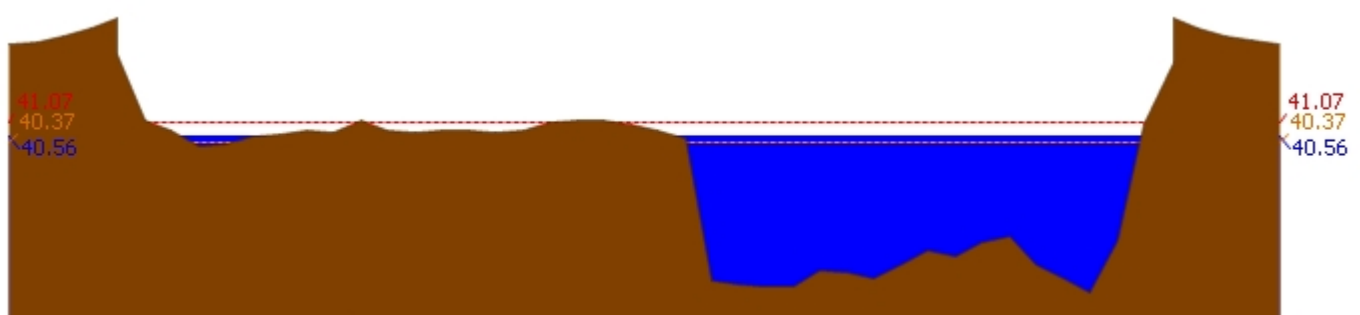
สถานี 060110T แม่น้ำปิงที่บ้านบางแก้ว ต.บางแก้ว อ.บรรพตพิสัย จ.นครสวรรค์ ระดับน้ำ 40.56 ม.รทก.
