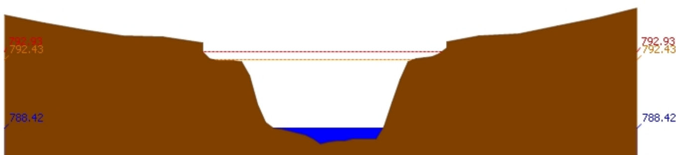
สถานี 061503T น้ำแม่ต้นที่บ้านคอย ต.ยางเปียง อ.อมก๋อย จ.เชียงใหม่ ระดับน้ำ 788.42 ม.รทก.
