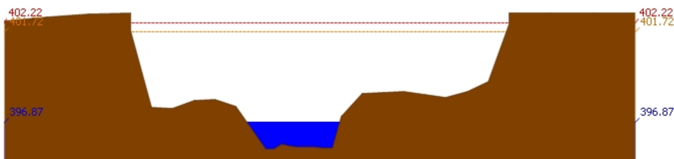
สถานี 060305T น้ำแม่จิดที่บ้านโป่งบัวบาน ต.แม่ปิง อ.พร้าว จ.เชียงใหม่ ระดับน้ำ 396.87 ม.รทก.
