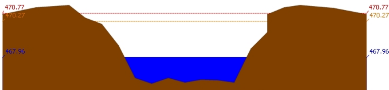
สถานี 061206T น้ำแม่แจ่มที่บ้านทัพ ต.ท่าผา อ.แม่แจ่ม จ.เชียงใหม่ ระดับน้ำ 467.96 ม.รทก.
