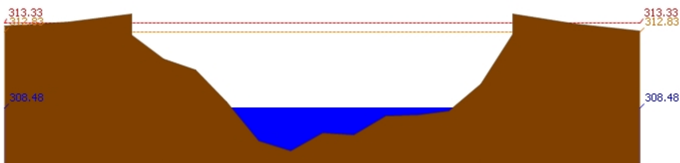
สถานี 060814T น้ำแม่ขานที่บ้านท่าโป่ง ต.บ้านแม อ.สันป่าตอง จ.เชียงใหม่ ระดับน้ำ 308.48 ม.รทก.
