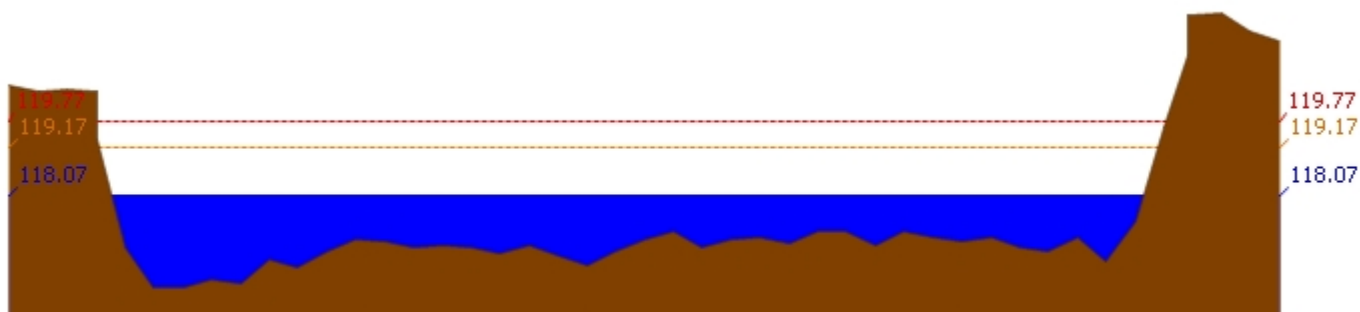
สถานี 060111T แม่น้ำปิงที่บ้านปากโรงห้วยจี้ ต.ตากออก อ.บ้านตาก จ.ตาก ระดับน้ำ 118.07 ม.รทก.
