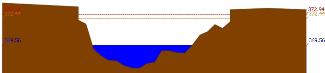
สถานี 060109T แม่น้ำปิงที่บ้านสบอ้อ ต.แม่ระ อ.เชียงดาว จ.เชียงใหม่ ระดับน้ำ 369.56 ม.รทก.
