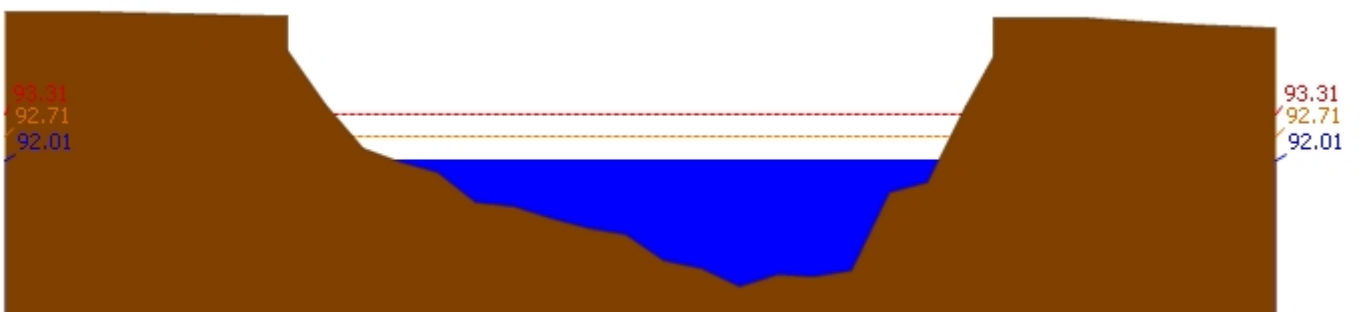
สถานี 061901T คลองแม่ระกาที่บ้านวังชะโอน ต.ท่าไม้ อ.พรานกระต่าย จ.กำแพงเพชร ระดับน้ำ 92.01 ม.รทก.
