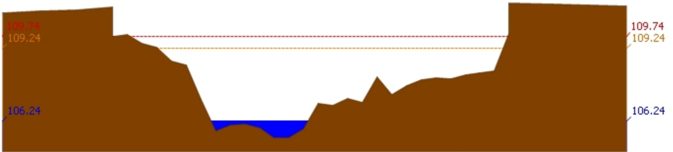
สถานี 061701T ฝายแม่ท้อที่อำเภอเมืองตาก ต.แม่ท้อ อ.เมืองตาก จ.ตาก ระดับน้ำ 106.24 ม.รทก.
