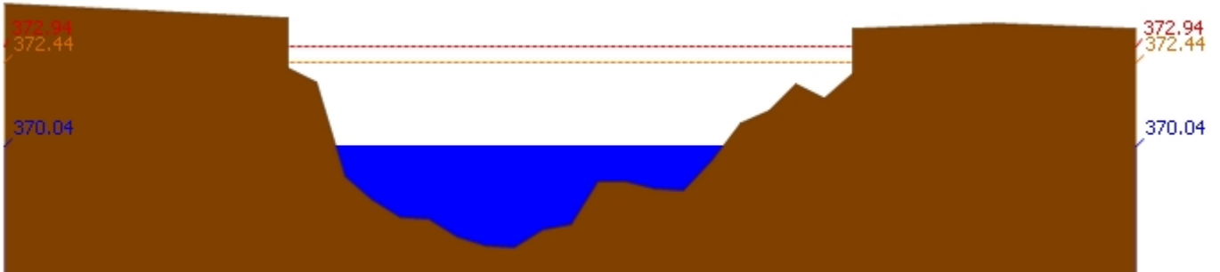
สถานี 060109T แม่น้ำปิงที่บ้านสบอ้อ ต.แม่ระ อ.เชียงดาว จ.เชียงใหม่ ระดับน้ำ 370.04 ม.รทก.
