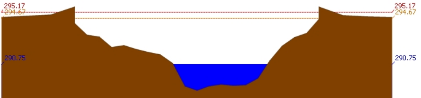
สถานี 060709T น้ำแม่กวังที่ลำพูน ต.เวียงยอง อ.เมือง จ.ลำพูน ระดับน้ำ 290.75 ม.รทก.
