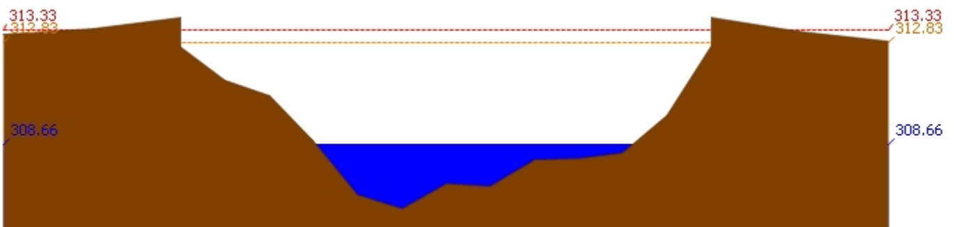
สถานี 060814T น้ำแม่ขานที่บ้านท่าโป่ง ต.บ้านแม อ.สันป่าตอง จ.เชียงใหม่ ระดับน้ำ 308.66 ม.รทก.
