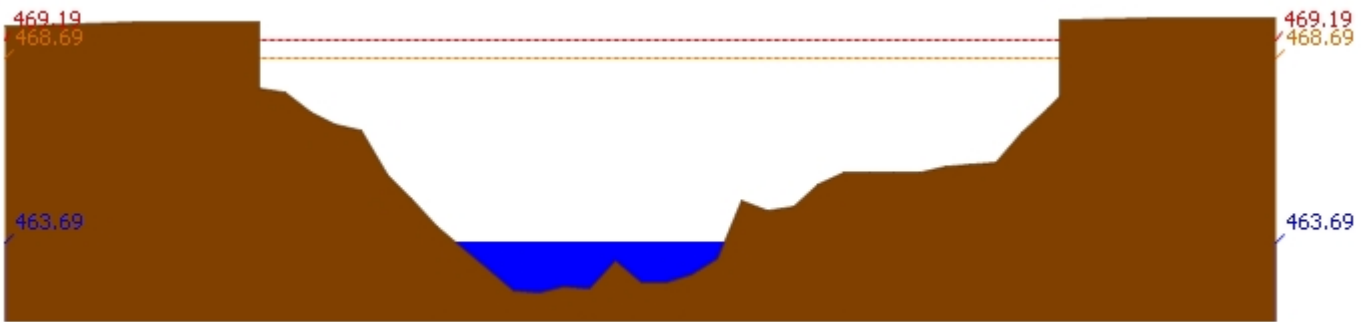
สถานี 060905T น้ำแม่ลี้ที่อำเภอลี้ ต.ลี้ อ.ลี้ จ.ลำพูน ระดับน้ำ 463.69 ม.รทก.
