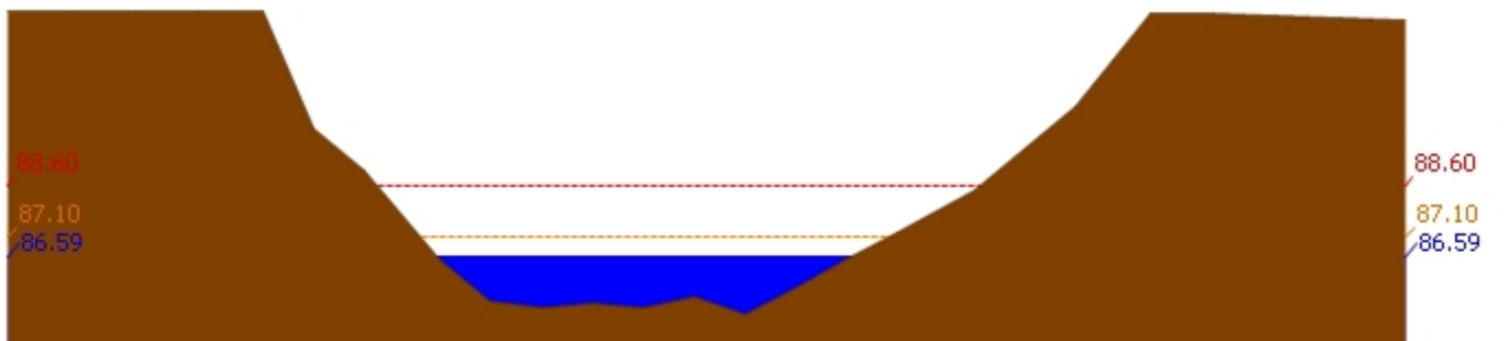
สถานี 120110T แม่น้ำป่าสักที่บ้านวังโบสถ์ ต.วังโบสถ์ อ.หนองไผ่ จ.เพชรบูรณ์ ระดับน้ำ 86.59 ม.รทก.
