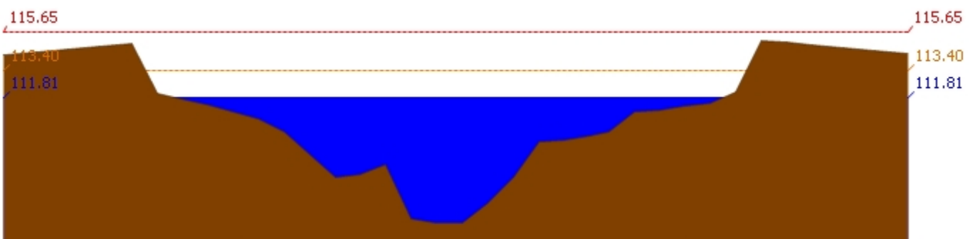
สถานี 120107T แม่น้ำป่าสักที่ อ.เมืองเพชรบูรณ์ ต.นาป่า อ.เมือง จ.เพชรบูรณ์ ระดับน้ำ 111.81 ม.รทก.
