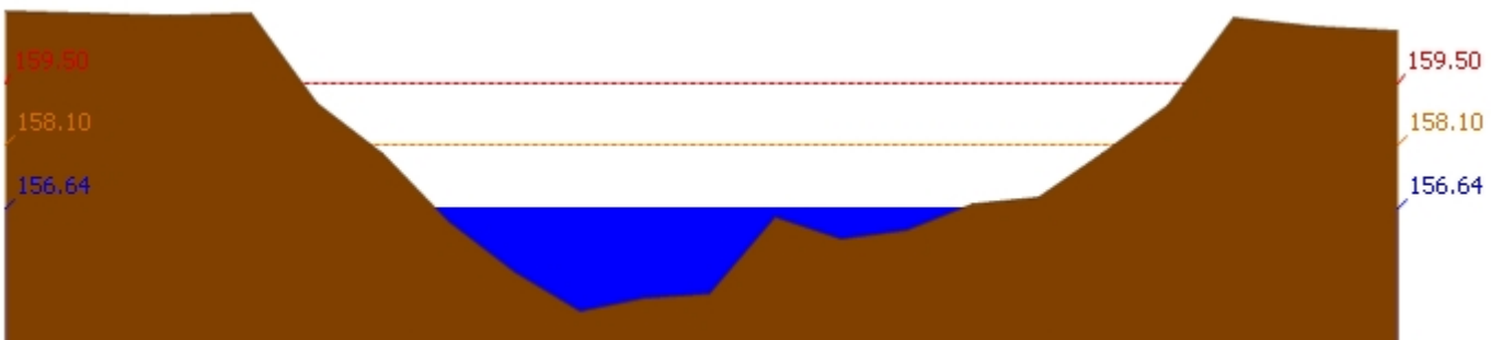
สถานี 120305T หัวน้ำพุที่ อ.หล่มเก่า ต.หล่มเก่า อ.หล่มเก่า จ.เพชรบูรณ์ ระดับน้ำ 156.64 ม.รทก.
