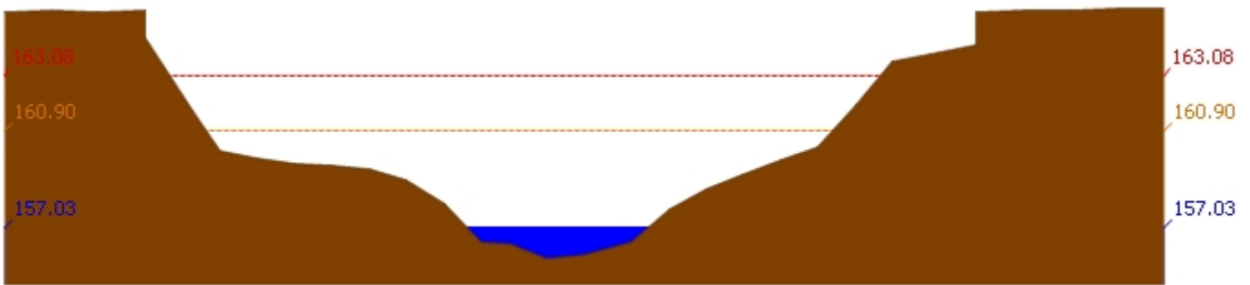
สถานี 120105T แม่น้ำป่าสักที่บ้านวังมเสหนือ ต.ท่าอิบุญ อ.หล่มสัก จ.เพชรบูรณ์ ระดับน้ำ 157.03 ม.รทก.
