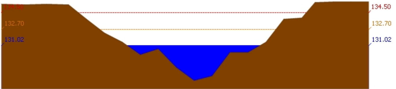
สถานี 120111T แม่น้ำป่าสักที่บ้านจางวาง ต.ลานบัว อ.หล่มสัก จ.เพชรบูรณ์ ระดับน้ำ 131.02 ม.รทก.
