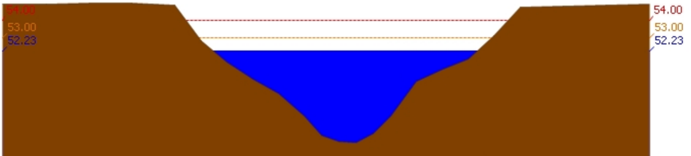
สถานี 120702T ลำสนธิที่บ้านท่าช้าง ต.หนองขาหย่าง อ.ชัยบาดาล จ.ลพบุรี ระดับน้ำ 52.23 ม.รทก.
