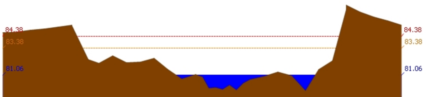
สถานี 062001T คลองสวนหมากที่บ้านน้ำไทรง ต.ท่าขุนราม อ.เมือง จ.กำแพงเพชร ระดับน้ำ 81.06 ม.รทก.
