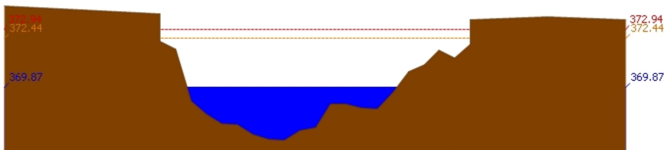
สถานี 060109T แม่น้ำปิงที่บ้านสบฮ้อ ต.แม่ระ อ.เชียงดาว จ.เชียงใหม่ ระดับน้ำ 369.87 ม.รทก.
