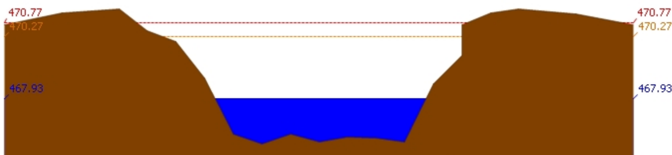
สถานี 061206T น้ำแม่แจ่มที่บ้านทัพ ต.ท่าผา อ.แม่แจ่ม จ.เชียงใหม่ ระดับน้ำ 467.93 ม.รทก.
