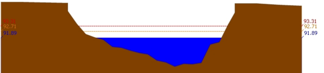
สถานี 061901T คลองแม่ระกาที่บ้านวังชะโอน ต.ท่าไม้ อ.พรานกระต่าย จ.กำแพงเพชร ระดับน้ำ 91.89 ม.รทก.
