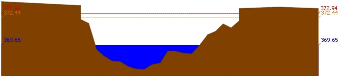
สถานี 060109T แม่ น้ำปิงที่บ้านสบอ้อ ต.แม่่นะ อ.เชียงดาว จ.เชียงใหม่ ระดับน้ำ 369.65 ม.รทก.
