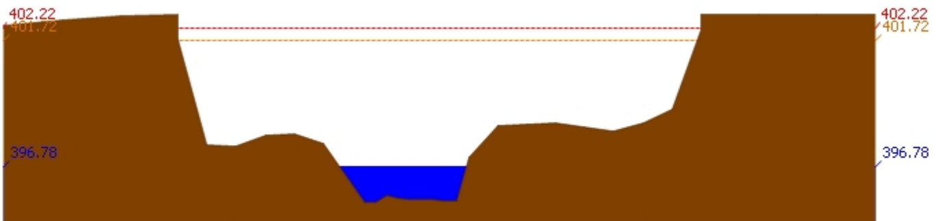
สถานี 060305T น้ำแม่จืดที่บ้านโป่งบัวบาน ต.แม่ป๋อง อ.พร้าว จ.เชียงใหม่ ระดับน้ำ 396.78 ม.รทก.
