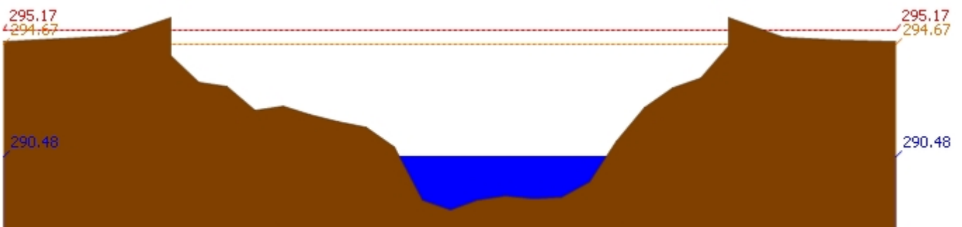
สถานี 060709T น้ำแม่กวงที่ลำพูน ต.เวียงยอง อ.เมือง จ.ลำพูน ระดับน้ำ 290.48 ม.รทก.
