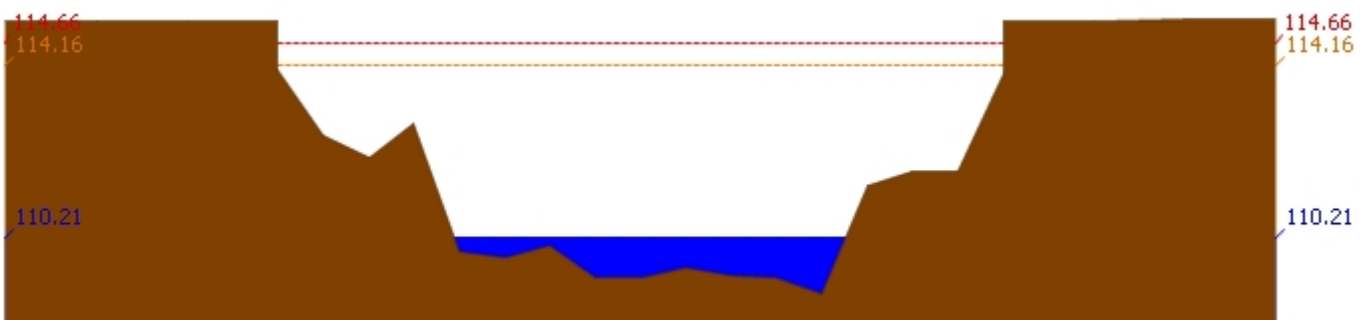
สถานี 061801T คลองวังเจ้าที่บ้านคลองลึก ต.เชียงทอง อ.วังเจ้า จ.ตาก ระดับน้ำ 110.21 ม.รทก.
