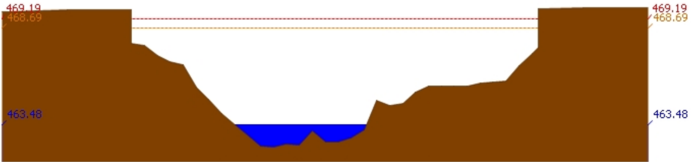
สถานี 060905T น้ำแม่สีที่อำเภอสีคิ้ว อ.สีคิ้ว จ.ลำพูน ระดับน้ำ 463.48 ม.รทก.
