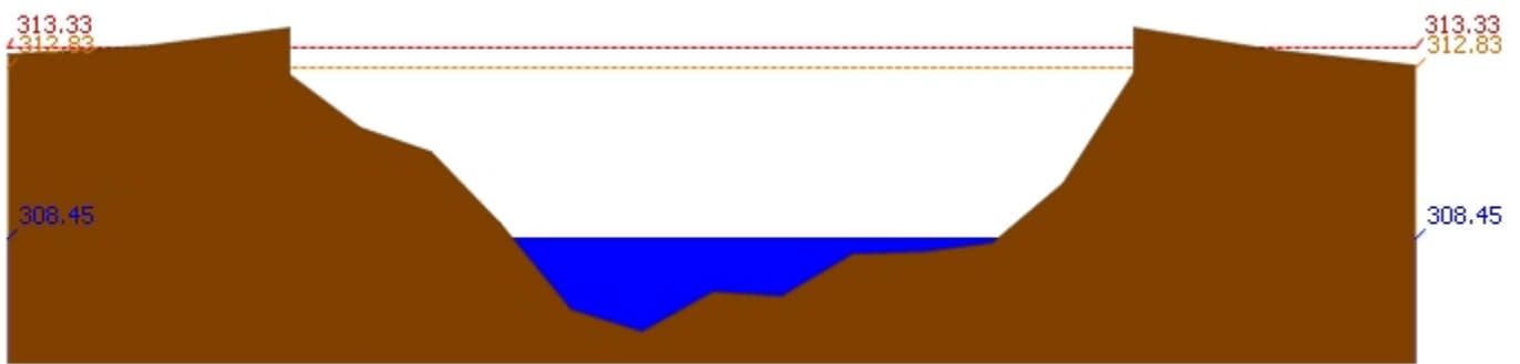
สถานี 060814T น้ำแม่ขานที่บ้านท่าโป่ง ต.บ้านแม อ.สันป่าตอง จ.เชียงใหม่ ระดับน้ำ 308.45 ม.รทก.
