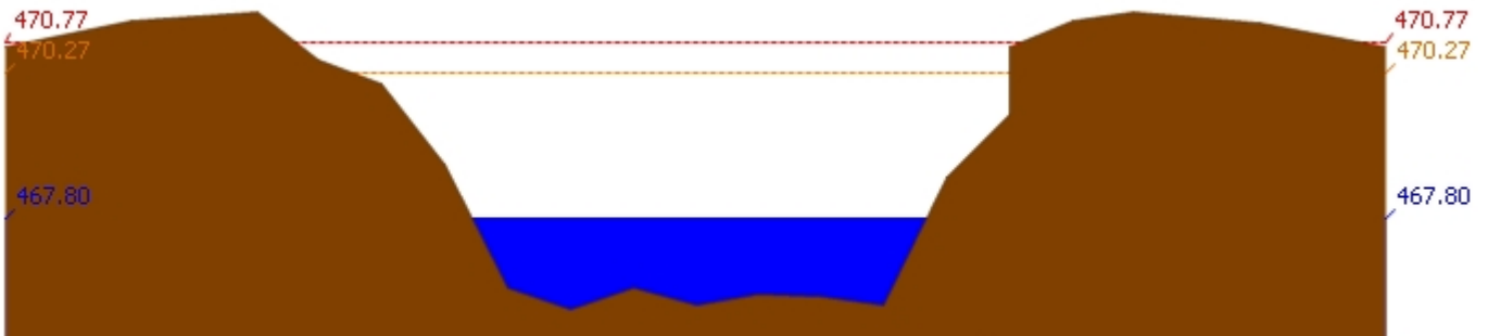
สถานี 061206T น้ำแม่แจ่มที่บ้านทัพ ต.ท่าผา อ.แม่แจ่ม จ.เชียงใหม่ ระดับน้ำ 467.80 ม.รทก.
