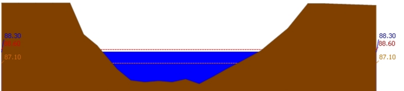
สถานี 120110T แม่น้ำป่าสักที่บ้านวังโบสถ์ ต.วังโบสถ์ อ.หนองไผ่ จ.เพชรบูรณ์ ระดับน้ำ 88.30 ม.รทก.
