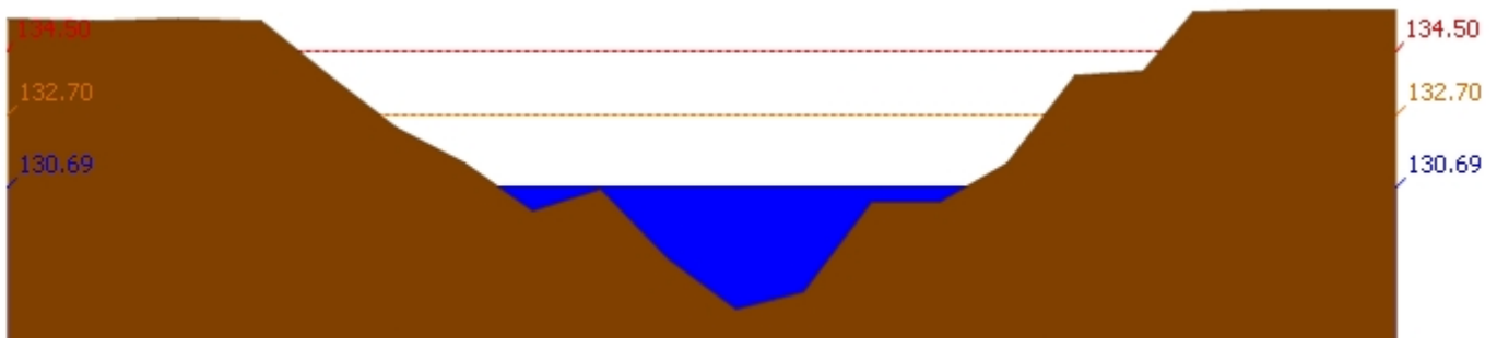
สถานี 120111T แม่น้ำป่าสักที่บ้านจางวาง ต.ลานบัว อ.หล่มสัก จ.เพชรบูรณ์ ระดับน้ำ 130.69 ม.รทก.
