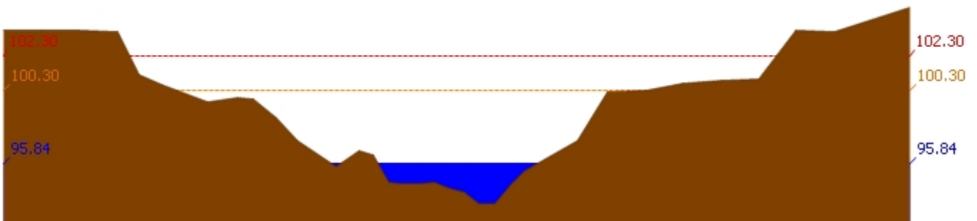
สถานี 120112T แม่น้ำป่าสักที่บ้านหนองแหวน ต.วังมะข่อ อ.เมือง จ.เพชรบูรณ์ ระดับน้ำ 95.84 ม.รทก.
