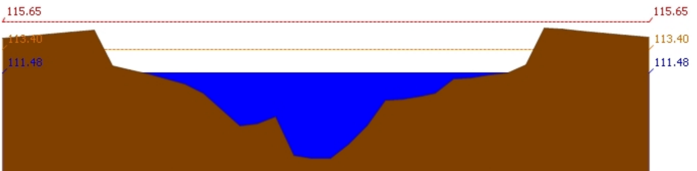
สถานี 120107T แม่น้ำป่าสักที่ อ.เมืองเพชรบูรณ์ ต.นาป่า อ.เมือง จ.เพชรบูรณ์ ระดับน้ำ 111.48 ม.รทก.
