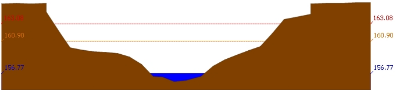
สถานี 120105T แม่น้ำป่าสักที่บ้านวังมเสหนือ ต.ท่าอิฐ อ.หล่มสัก จ.เพชรบูรณ์ ระดับน้ำ 156.77 ม.รทก.
