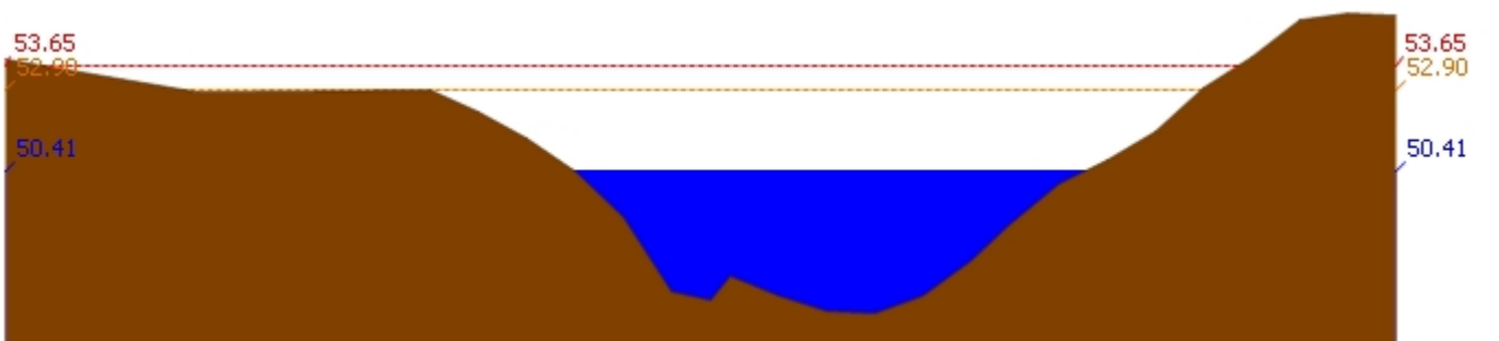
สถานี 120113T แม่น้ำป่าสักที่บ้านเขาค้าง ต.คลองกระจิง อ.ศรีเทพ จ.เพชรบูรณ์ ระดับน้ำ 50.41 ม.รทก.
