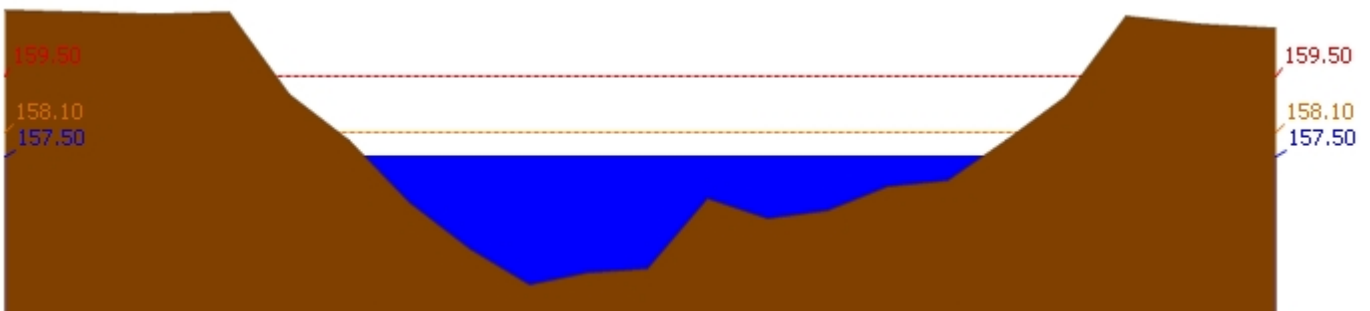
สถานี 120305T หัวน้ำพุที่ อ.หล่มเก่า ต.หล่มเก่า อ.หล่มเก่า จ.เพชรบูรณ์ ระดับน้ำ 157.50 ม.รทก.
