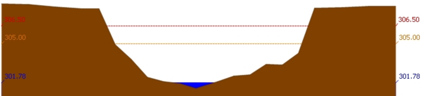
สถานี 120304T หัวน้ำพุที่บ้านกกกะบาก ต.โป่ง อ.ด่านซ้าย จ.เลย ระดับน้ำ 301.78 ม.รทก.
