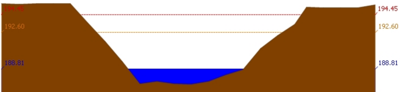
สถานี 120901T ห้วยมวกเหล็กที่ อ.มวกเหล็ก ต.มวกเหล็ก อ.มวกเหล็ก จ.สระบุรี ระดับน้ำ 188.81 ม.รทก.
