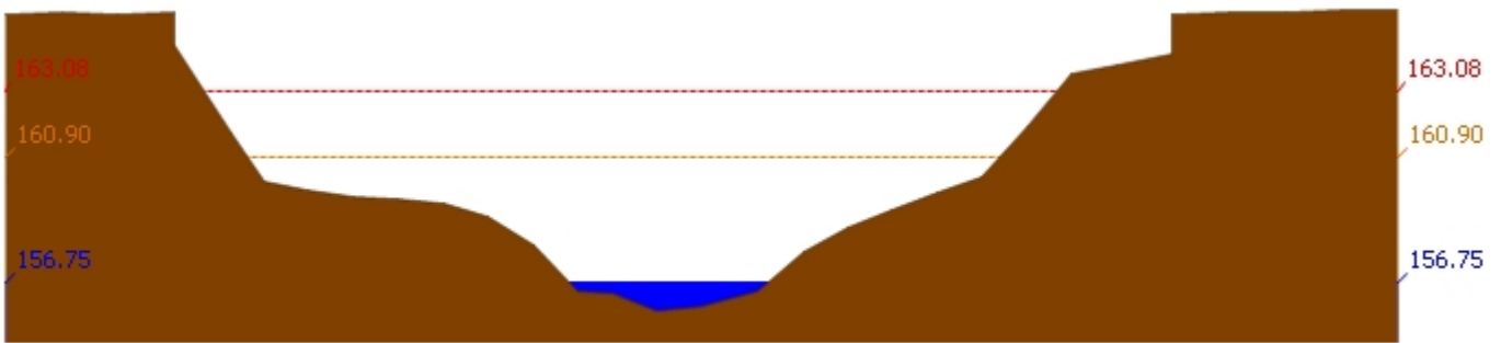
สถานี 120105T แม่น้ำป่าสักที่บ้านวังมเสหนือ ต.ท่าอิบุญ อ.หล่มสัก จ.เพชรบูรณ์ ระดับน้ำ 156.75 ม.รทก.
