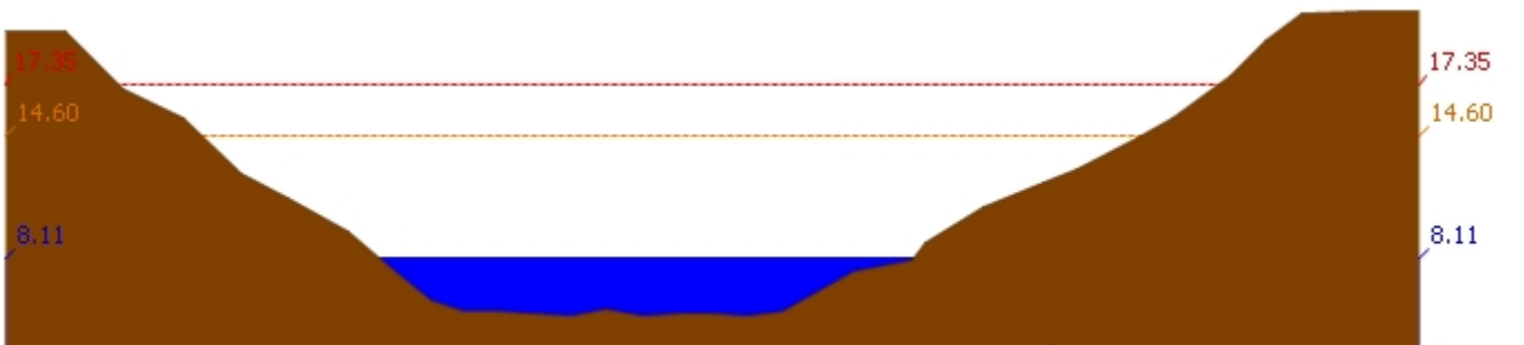
สถานี 120109T แม่น้ำป่าสักที่ อ.แก่งคอย ต.แก่งคอย อ.แก่งคอย จ.สระบุรี ระดับน้ำ 8.11 ม.รทก.
