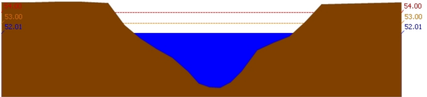
สถานี 120702T ลำสนธิที่บ้านท่าช้าง ต.หนองขาหย่าง อ.ชัยบาดาล จ.ลพบุรี ระดับน้ำ 52.01 ม.รทก.
