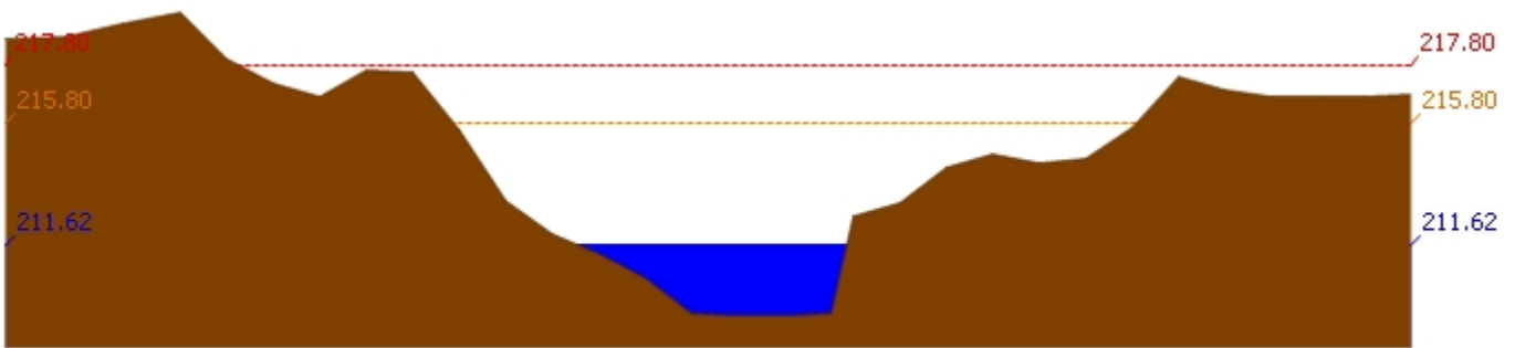
สถานี 120205T แม่น้ำป่าสักที่บ้านอู่กะทาด ต.ศิลา อ.หล่มเก่า จ.เพชรบูรณ์ ระดับน้ำ 211.62 ม.รทก.
