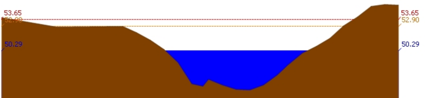
สถานี 120113T แม่น้ำป่าสักที่บ้านเขาค้าง ต.คลองกระจิง อ.ศรีเทพ จ.เพชรบูรณ์ ระดับน้ำ 50.29 ม.รทก.
