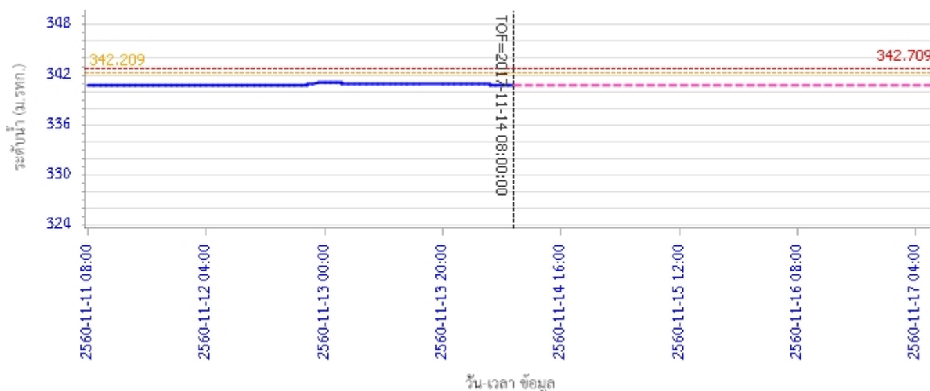
ผลการคำนวณระดับน้ำ สถานี 070304T น้ำแม่สอยที่บ้านหนองกอก ต.แม่สวก อ.แจ้ห่ม จ.ลำปาง
