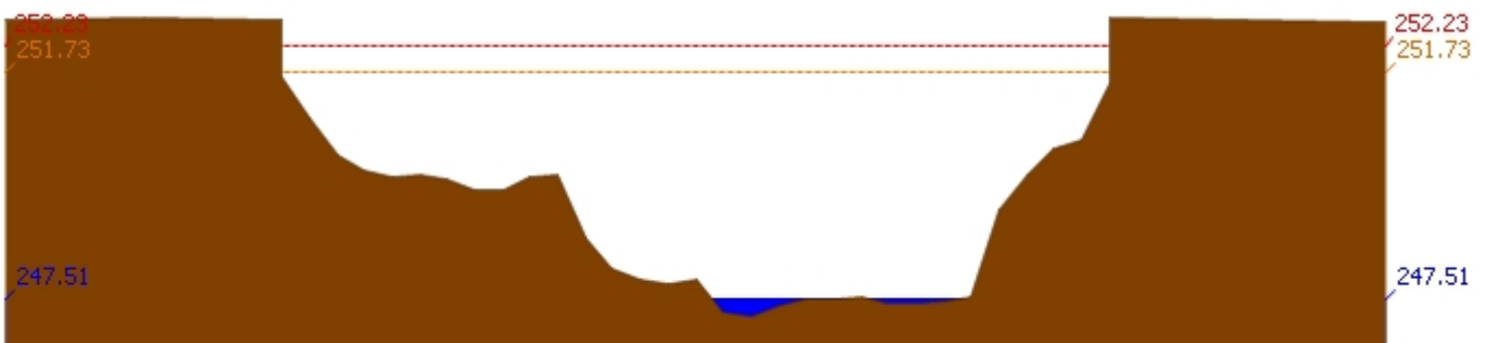
สถานี 070403T น้ำแม่คู่ที่บ้านแค้ ต.บ้านเป้า อ.เมืองลำปาง จ.ลำปาง ระดับน้ำ 247.51 ม.รทก.
