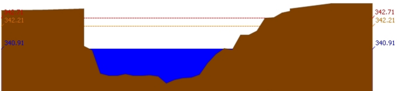
สถานี 070304T น้ำแม่สอยที่บ้านหนองกอก ต.แม่สอก อ.แจ้ห่ม จ.ลำปาง ระดับน้ำ 340.91 ม.รทก.
