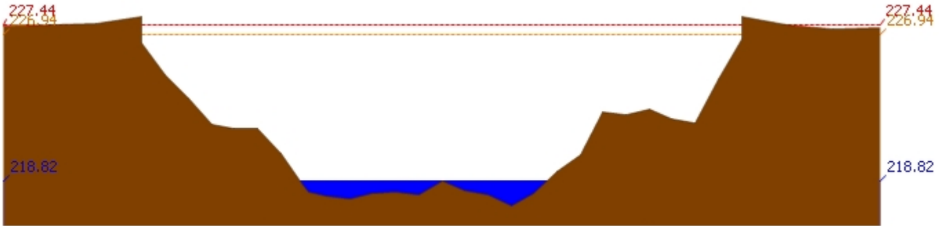
สถานี 070113T แม่น้ำวังที่ จ.ลำปาง ต.เวียงเหนือ อ.เมืองลำปาง จ.ลำปาง ระดับน้ำ 218.82 ม.รทก.
