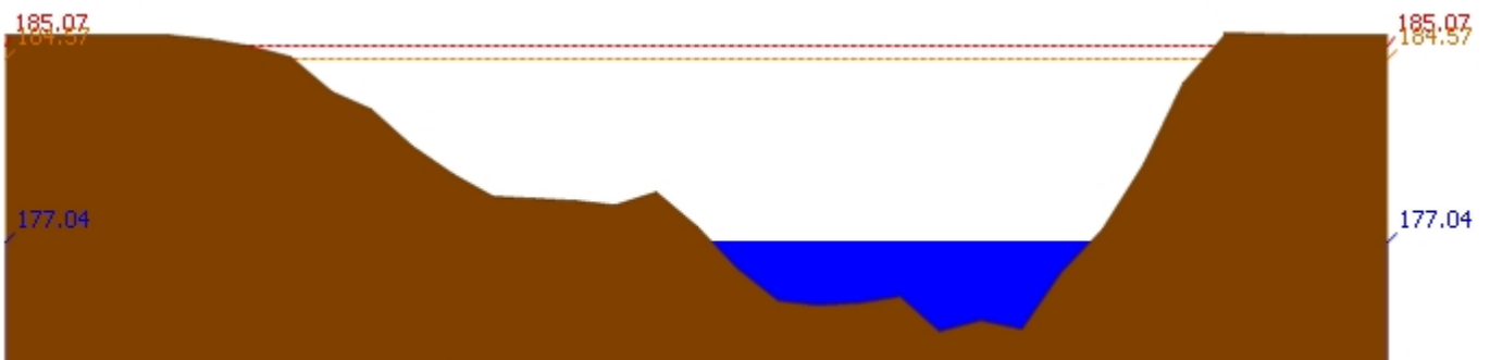
สถานี 070116T แม่น้ำวังที่บ้านแม่เตี๊ยะ ต.แม่ถอด อ.เถิน จ.ลำปาง ระดับน้ำ 177.04 ม.รทก.
