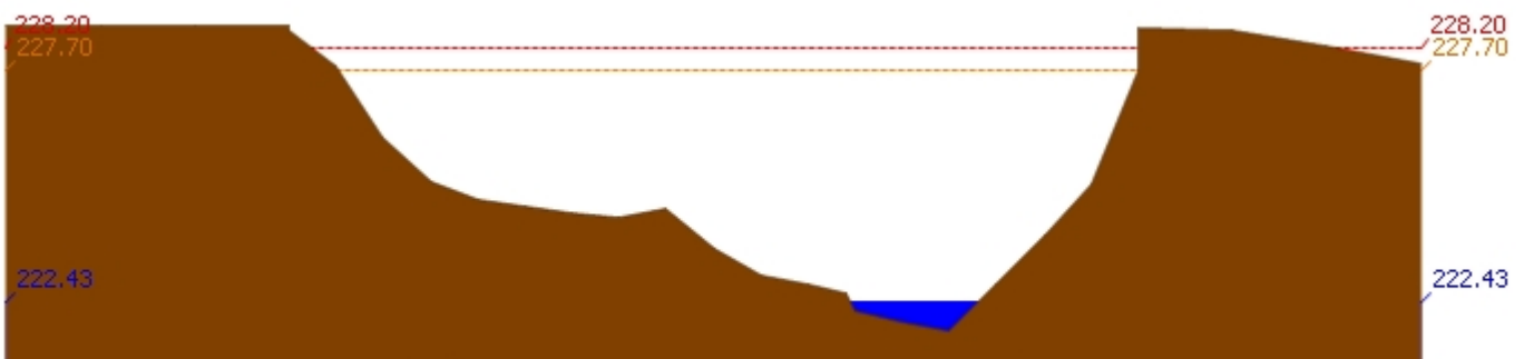
สถานี 070703T น้ำแม่คำที่บ้านนาบอน ต.ทุ่งงาม อ.เสริมงาม จ.ลำปาง ระดับน้ำ 222.43 ม.รทก.
