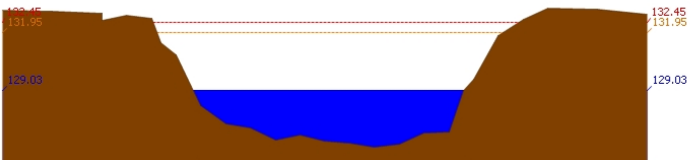
สถานี 070118T แม่น้ำวังที่บ้านแม่สลิด ต.แม่สลิด อ.บ้านตาก จ.ตาก ระดับน้ำ 129.03 ม.รทก.
