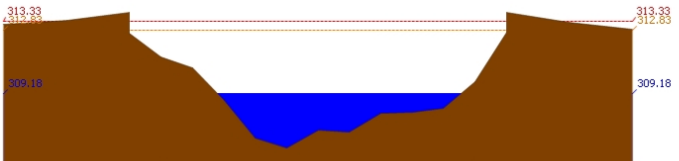
สถานี 060814T น้ำแม่ขานที่บ้านท่าโป่ง ต.บ้านแม อ.สันป่าตอง จ.เชียงใหม่ ระดับน้ำ 309.18 ม.รทก.
