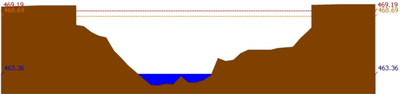
สถานี 060905T น้ำแม่ลี้ที่อำเภอลี้ ต.ลี้ อ.ลี้ จ.ลำพูน ระดับน้ำ 463.36 ม.รทก.
