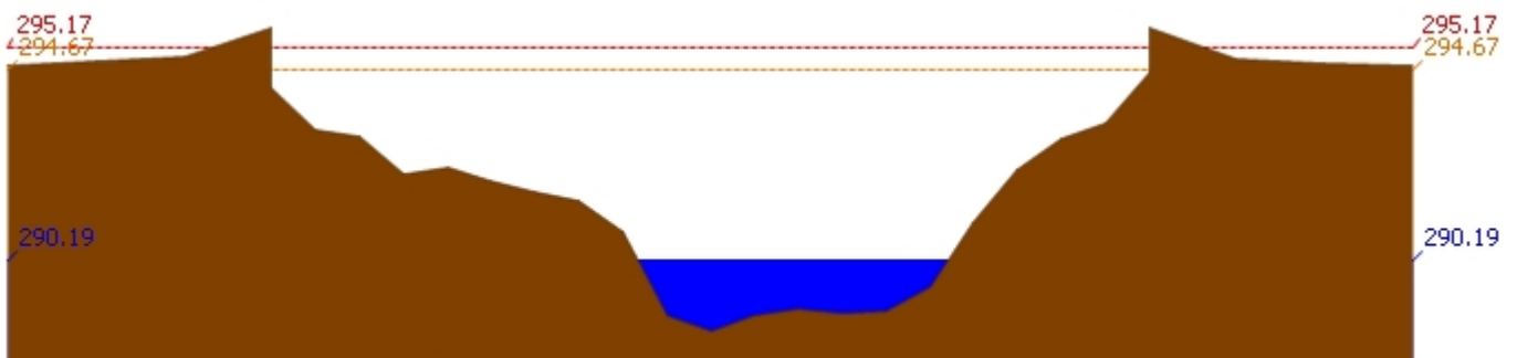
สถานี 060709T น้ำแม่กวังที่ลำพูน ต.เวียงยอง อ.เมือง จ.ลำพูน ระดับน้ำ 290.19 ม.รทก.
