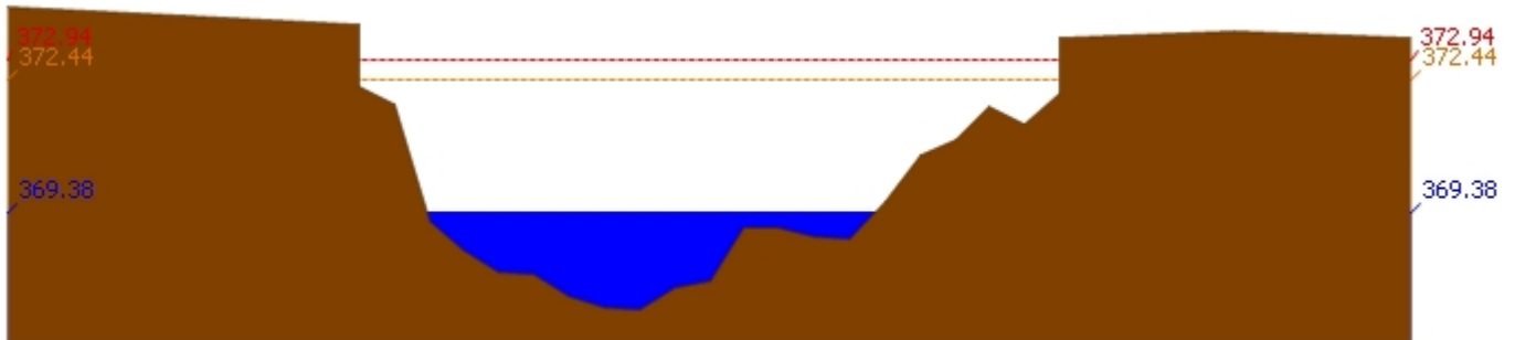
สถานี 060109T แม่น้ำปิงที่บ้านสบอ้อ ต.แม่่นะ อ.เชียงดาว จ.เชียงใหม่ ระดับน้ำ 369.38 ม.รทก.
