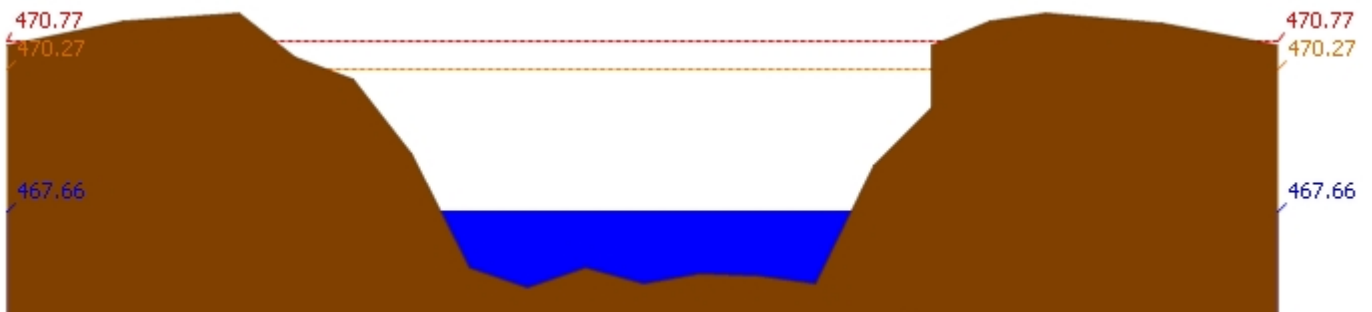
สถานี 061206T น้ำแม่แจ่มที่บ้านทัพ ต.ท่าผา อ.แม่แจ่ม จ.เชียงใหม่ ระดับน้ำ 467.66 ม.รทก.
