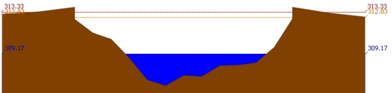
สถานี 060814T น้ำแม่ฆานที่บ้านท่าโป่ง ต.บ้านแม อ.สันป่าตอง จ.เชียงใหม่ ระดับน้ำ 309.17 ม.รทก.
