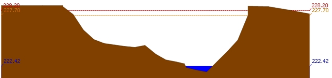
สถานี 070703T น้ำแม่ตำที่บ้านนาบอน ต.ทุ่งงาม อ.เสริมงาม จ.ลำปาง ระดับน้ำ 222.42 ม.รทก.
