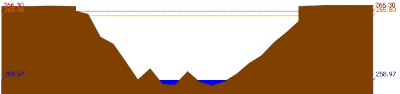
สถานี 070604T น้ำแม่จางที่บ้านสุโหมโขมมงคล ต.หัวเสือ อ.แม่ทะ จ.ลำปาง ระดับน้ำ 258.97 ม.รทก.
