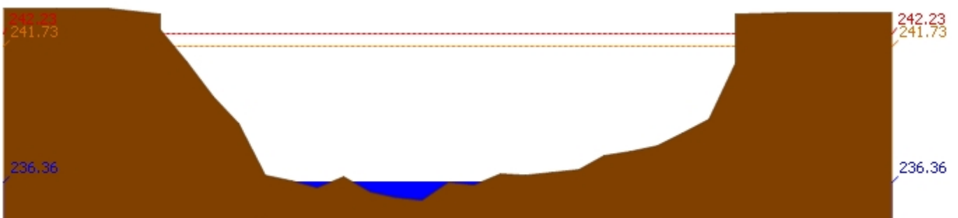
สถานี 070114T แม่น้ำวังที่บ้านปงชัย ต.บ้านเสด็จ อ.เมืองลำปาง จ.ลำปาง ระดับน้ำ 236.36 ม.รทก.
