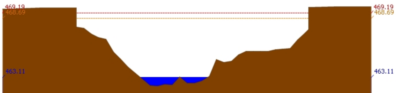
สถานี 060905T น้ำแม่ลี้ที่อำเภอลี้ ต.ลี้ อ.ลี้ จ.ลำพูน ระดับน้ำ 463.11 ม.รทก.
