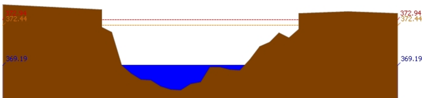
สถานี 060109T แม่น้ำปิงที่บ้านสบฮ้อย ต.แม่ระ อ.เชียงดาว จ.เชียงใหม่ ระดับน้ำ 369.19 ม.รทก.
