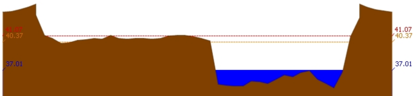
สถานี 060110T แม่น้ำปิงที่บ้านบางแก้ว ต.บางแก้ว อ.บรรพตพิสัย จ.นครสวรรค์ ระดับน้ำ 37.01 ม.รทก.
