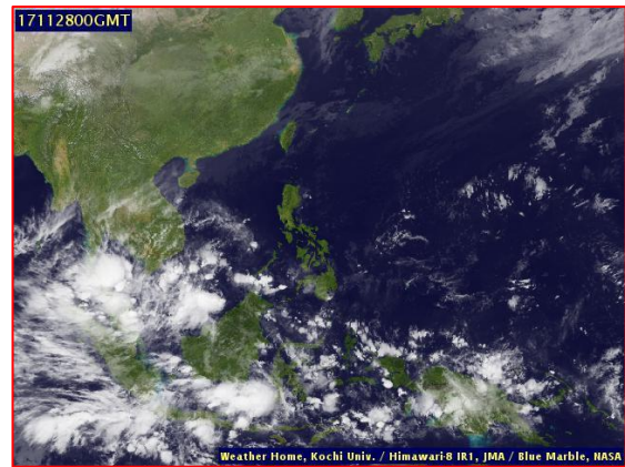
ภาพถ่ายจากดาวเทียม วันที่ 28 พ.ย. 2560 เวลา 07.00 น.
