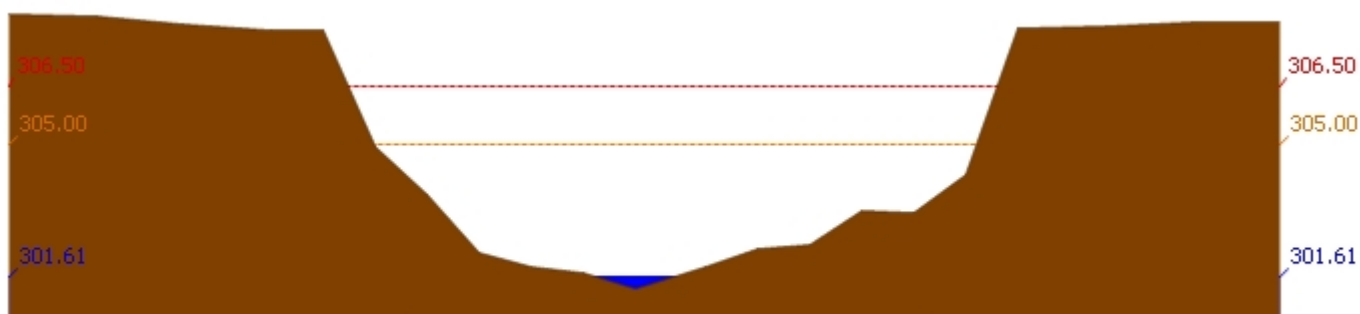
สถานี 120304T ห้วยน้ำพุที่บ้านกกกะบาก ต.โป่ง อ.ด่านซ้าย จ.เลย ระดับน้ำ 301.61 ม.รทก.
