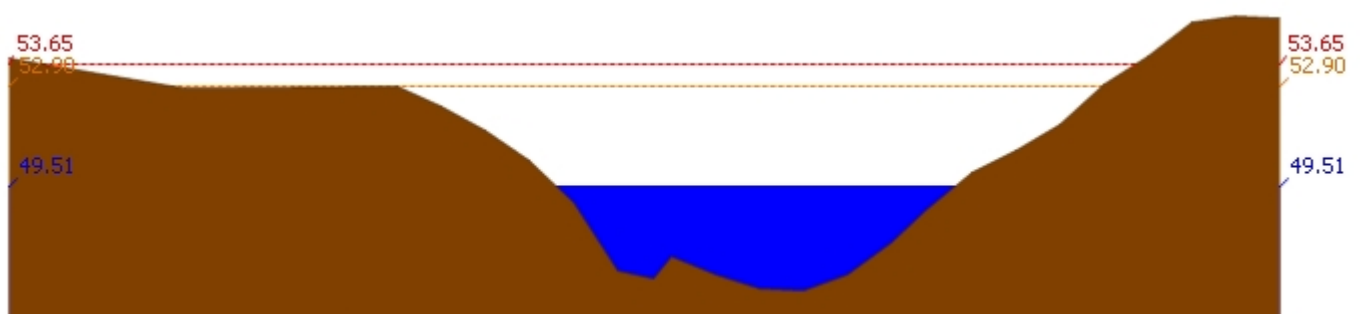
สถานี 120113T แม่น้ำป่าสักที่บ้านเขาค้าง ต.คลองกระจิง อ.ศรีเทพ จ.เพชรบูรณ์ ระดับน้ำ 49.51 ม.รทก.
