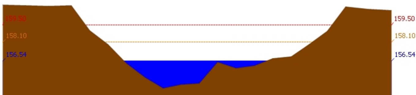
สถานี 120305T ห้วยน้ำพุที่ อ.หล่มเก่า ต.หล่มเก่า อ.หล่มเก่า จ.เพชรบูรณ์ ระดับน้ำ 156.54 ม.รทก.
