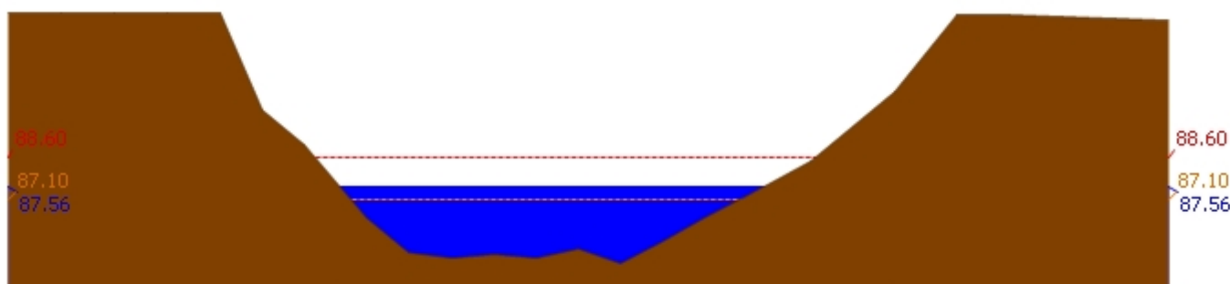
สถานี 120110T แม่น้ำป่าสักที่บ้านวังโบสถ์ ต.วังโบสถ์ อ.หนองไผ่ จ.เพชรบูรณ์ ระดับน้ำ 87.56 ม.รทก.
