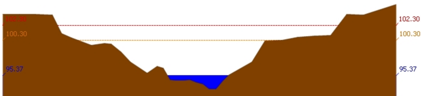
สถานี 120112T แม่น้ำป่าสักที่บ้านหนองแหวน ต.วังมะข่อ อ.เมือง จ.เพชรบูรณ์ ระดับน้ำ 95.37 ม.รทก.
