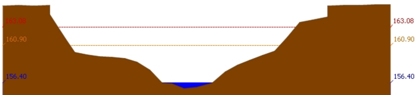
สถานี 120105T แม่น้ำป่าสักที่บ้านวังมสเหนือ ต.ทำอินดู อ.หล่มสัก จ.เพชรบูรณ์ ระดับน้ำ 156.40 ม.รทก.
