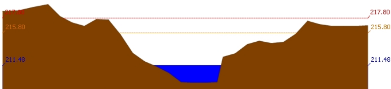
สถานี 120205T แม่น้ำป่าสักที่บ้านอุ้มกะทาด ต.ศิลา อ.หล่มเก่า จ.เพชรบูรณ์ ระดับน้ำ 211.48 ม.รทก.
