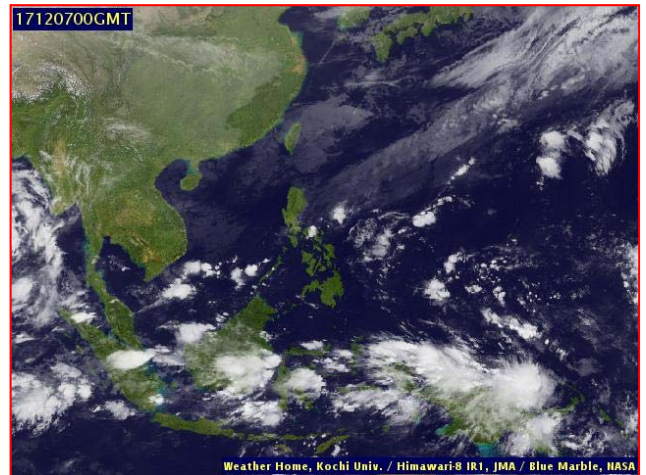
ภาพถ่ายจากดาวเทียม วันที่ ๗ ธ.ค. ๒๕๖๐ เวลา ๐๗.๐๐ น.
