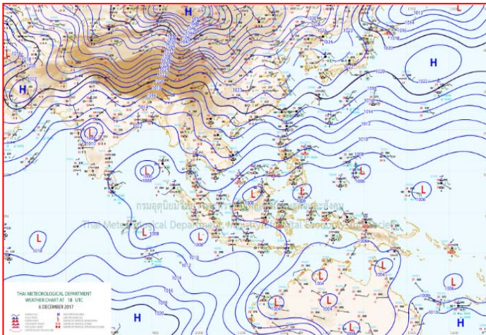
แผนที่อากาศ วันที่ ๗ ธ.ค. ๒๕๖๐ เวลา ๐๑.๐๐ น.
