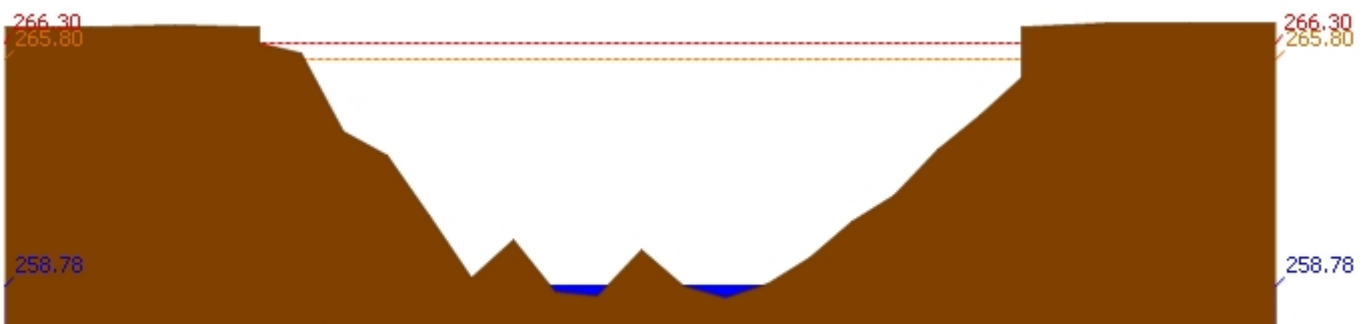
สถานี 070604T น้ำแม่จางที่บ้านสุใหม่โขมยมงคล ต.หัวเสือ อ.แม่ทะ จ.ลำปาง ระดับน้ำ 258.78 ม.รทก.
