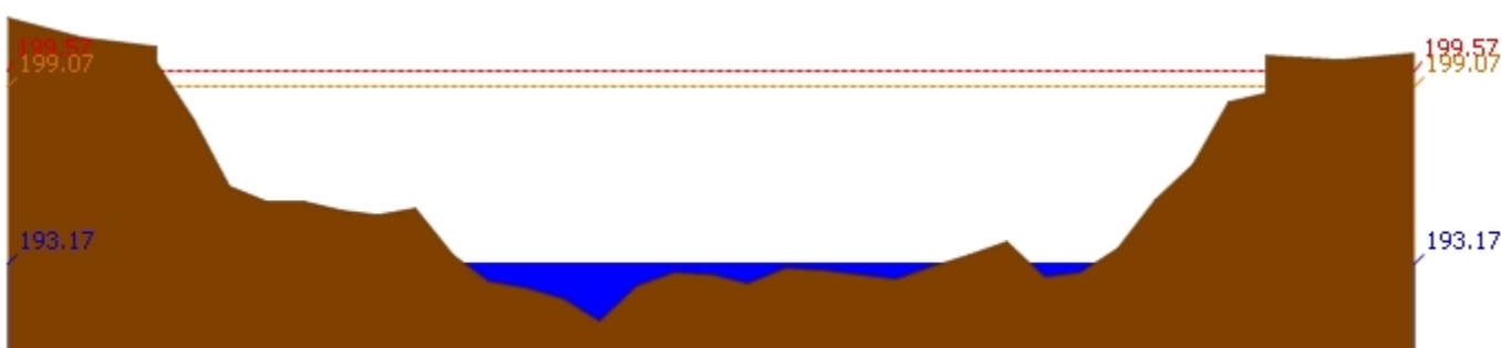
สถานี 070115T น้ำแม่วังที่บ้านอ้อ ต.แม่แก้ว อ.สบปราบ จ.ลำปาง ระดับน้ำ 193.17 ม.รทก.
