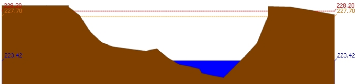
สถานี 070703T น้ำแม่คำที่บ้านนาบอน ต.ทุ่งงาม อ.เสริมงาม จ.ลำปาง ระดับน้ำ 223.42 ม.รทก.
