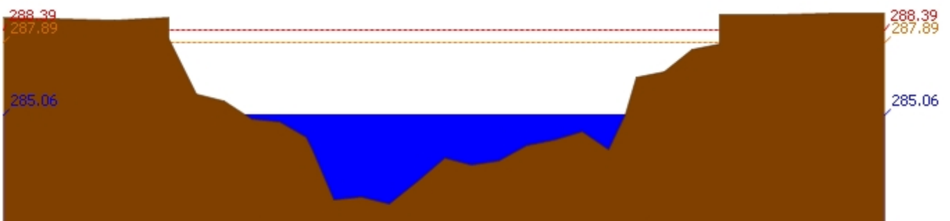
สถานี 070111T แม่น้ำวังที่บ้านโป่งชัย ต.บ้านเสา อ.แจ้ห่ม จ.ลำปาง ระดับน้ำ 285.06 ม.รทก.
